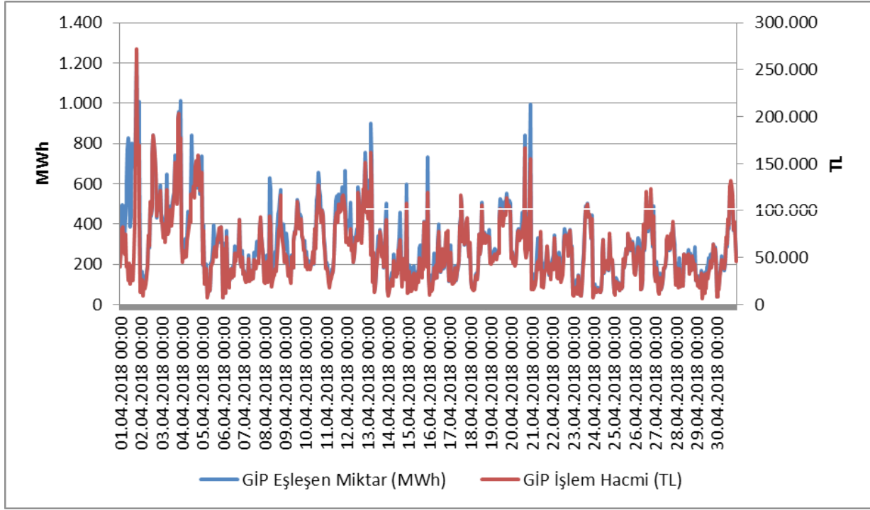
Şekil 4.10 Nisan 2018 Döneminde Gün İçi Piyasası (GİP) İşlem Hacminin Saatlik Gelişimi (TL-MWh)
