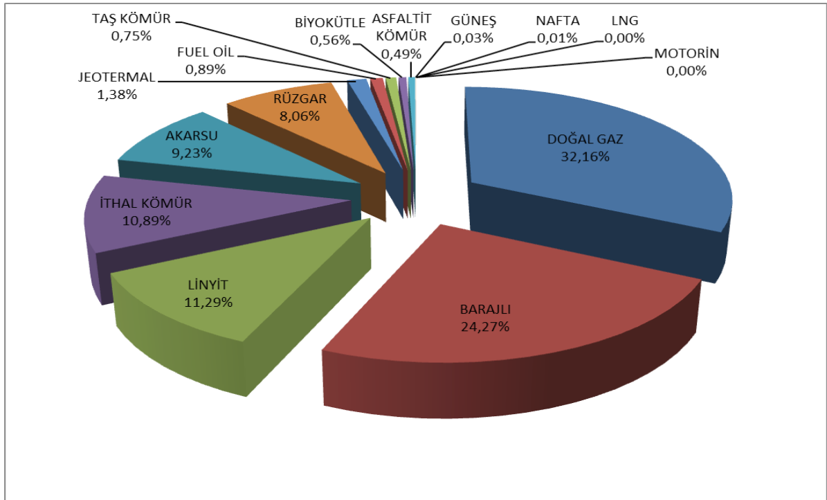
Şekil 1.2 2018 Yılı Nisan Ayı Sonu İtibariyle Lisanslı Elektrik Kurulu Gücünün Kaynak Bazında Dağılımı (%)
