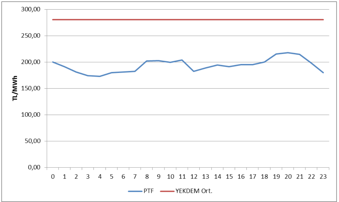
Şekil 1.13 Nisan 2018 Döneminde YEKDEM Aylık Ortalama Fiyatı ile Piyasa Takas Fiyatının (PTF) Saatlik Dağılımı (TL/MWh)
