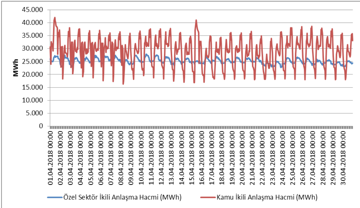
Şekil 4.13 Nisan 2018 Döneminde İkili Anlaşma Hacminin Saatlik Gelişimi (MWh)
