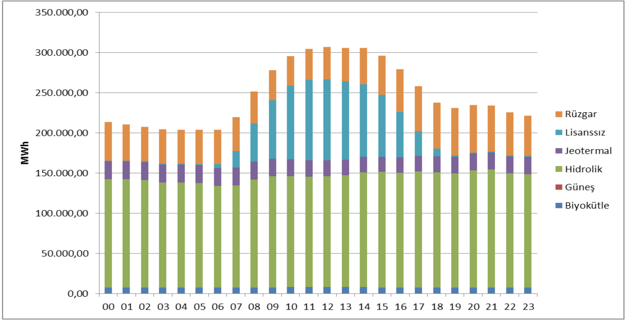
Şekil 1.11 Nisan 2018 Döneminde YEKDEM Kapsamındaki Üretim Saatlik Bazda Kaynaklara Göre Dağılımı (MWh)
