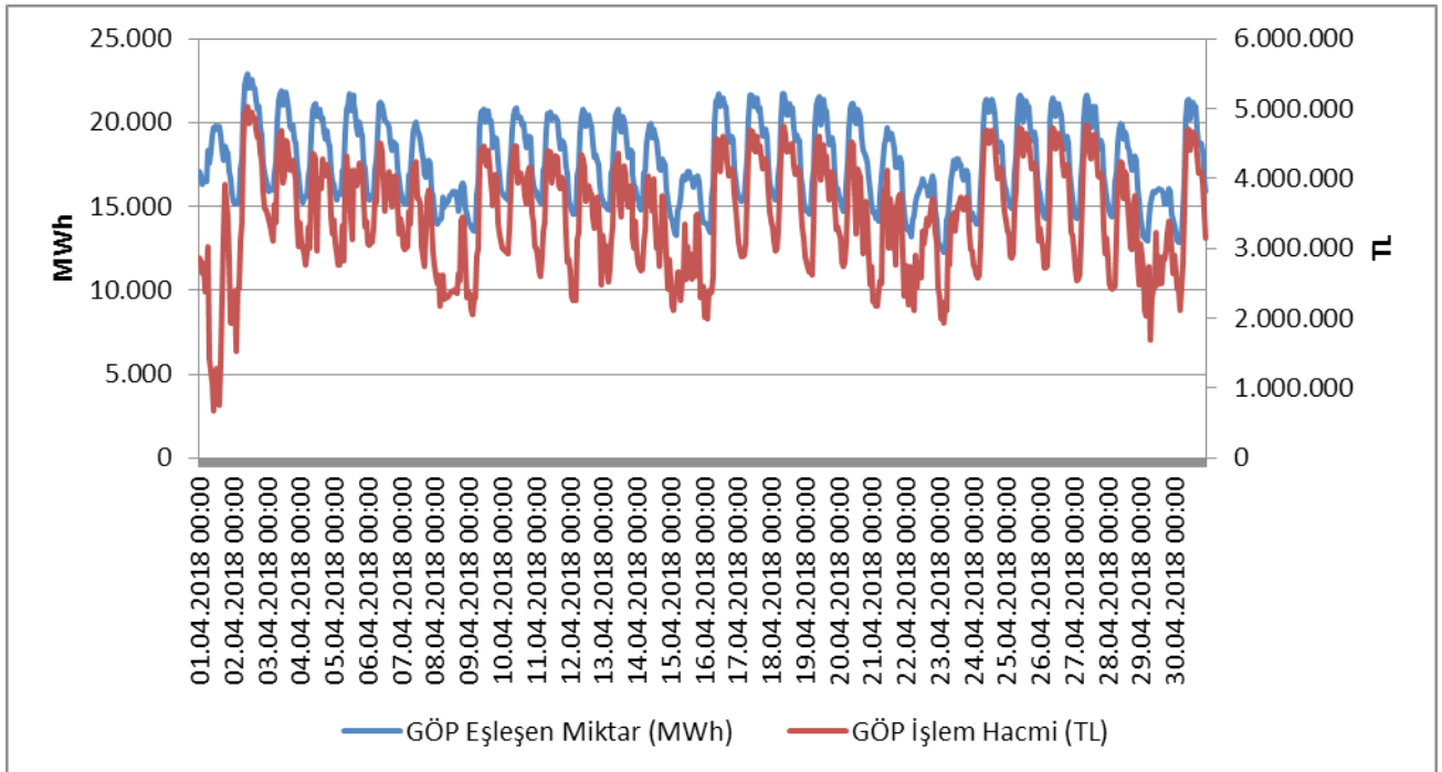
Şekil 4.2 Nisan 2018 Döneminde Gün Öncesi Piyasası (GÖP) İşlem Hacminin Saatlik Gelişimi (TL-MWh)
