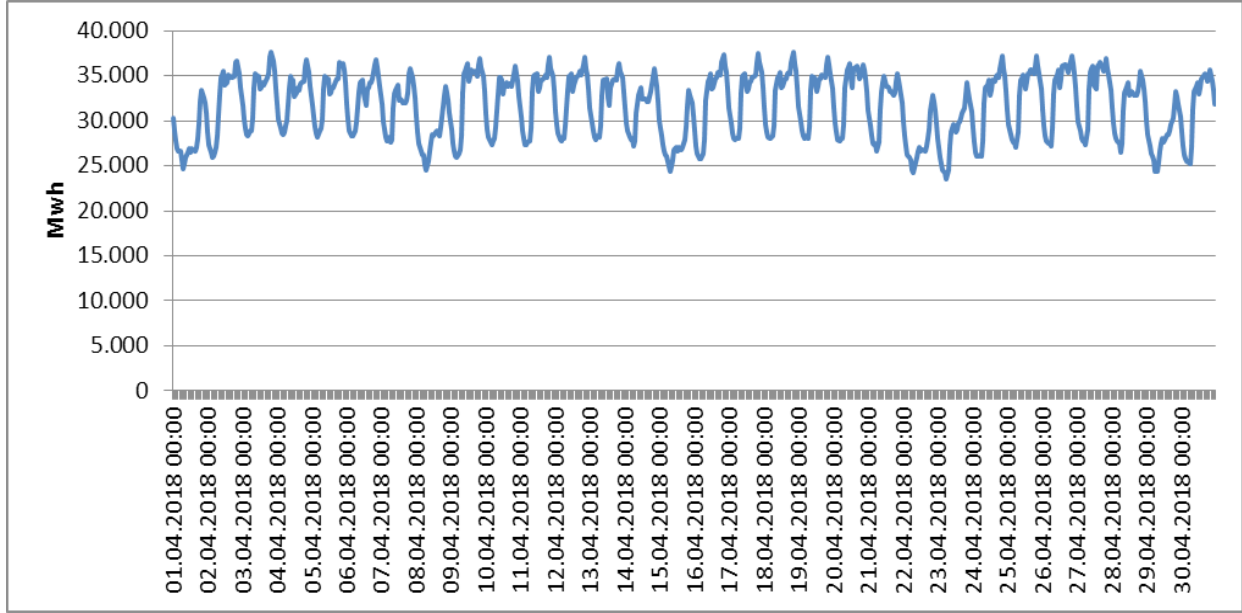
Şekil 2.1. Nisan 2018 Döneminde Elektrik Tüketiminin Saatlik Gelişimi (MWh)
