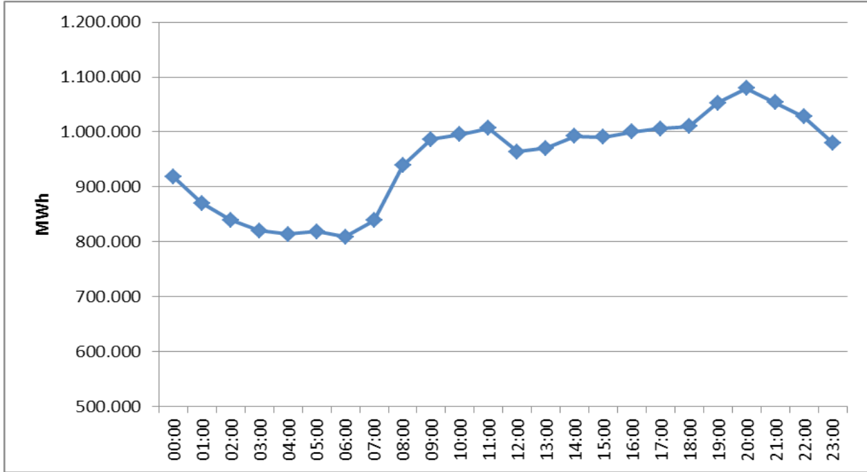
Şekil 2.2. Nisan 2018 Döneminde Elektrik Tüketiminin Saat Bazında Dağılımı (MWh)
