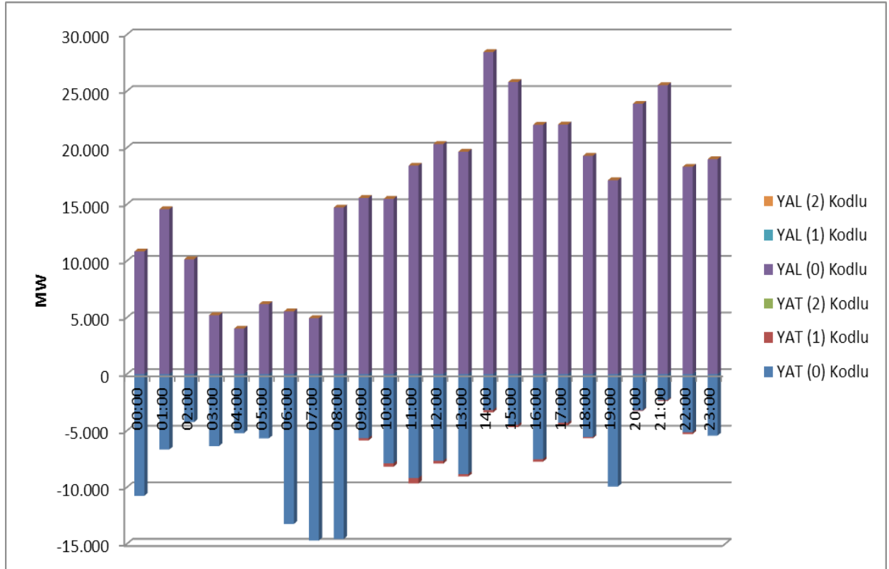
Şekil 4.7 Nisan 2018 Döneminde Dengeleme Güç Piyasasında (DGP) Verilen Talimatların Saatlik Bazda Dağılımı (MW)
