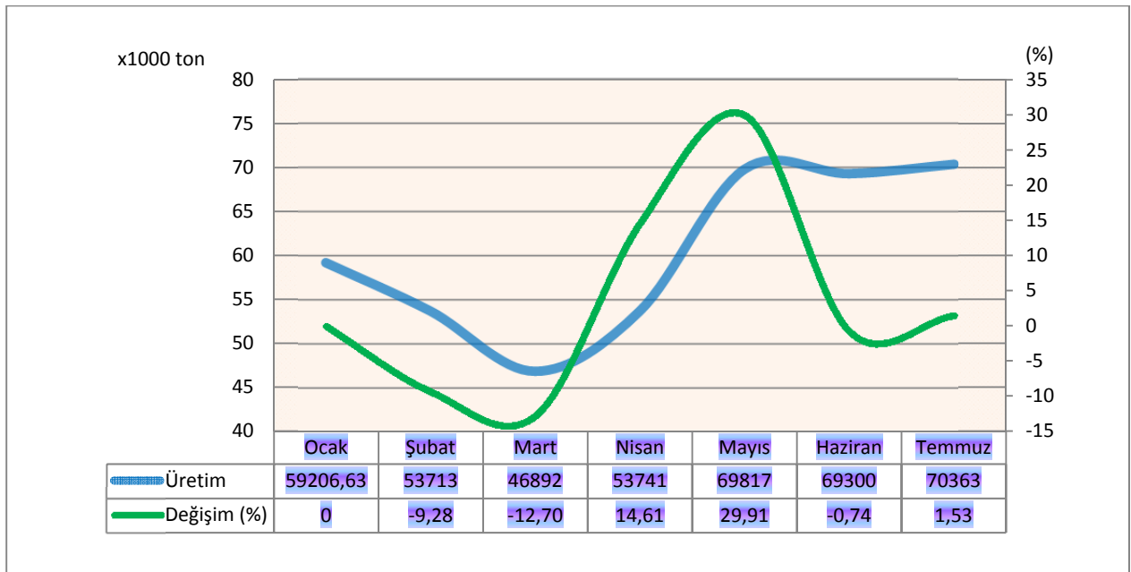
Şekil 3.1.1: 2013 yılı aylık LPG üretim miktarı ve değişimi
