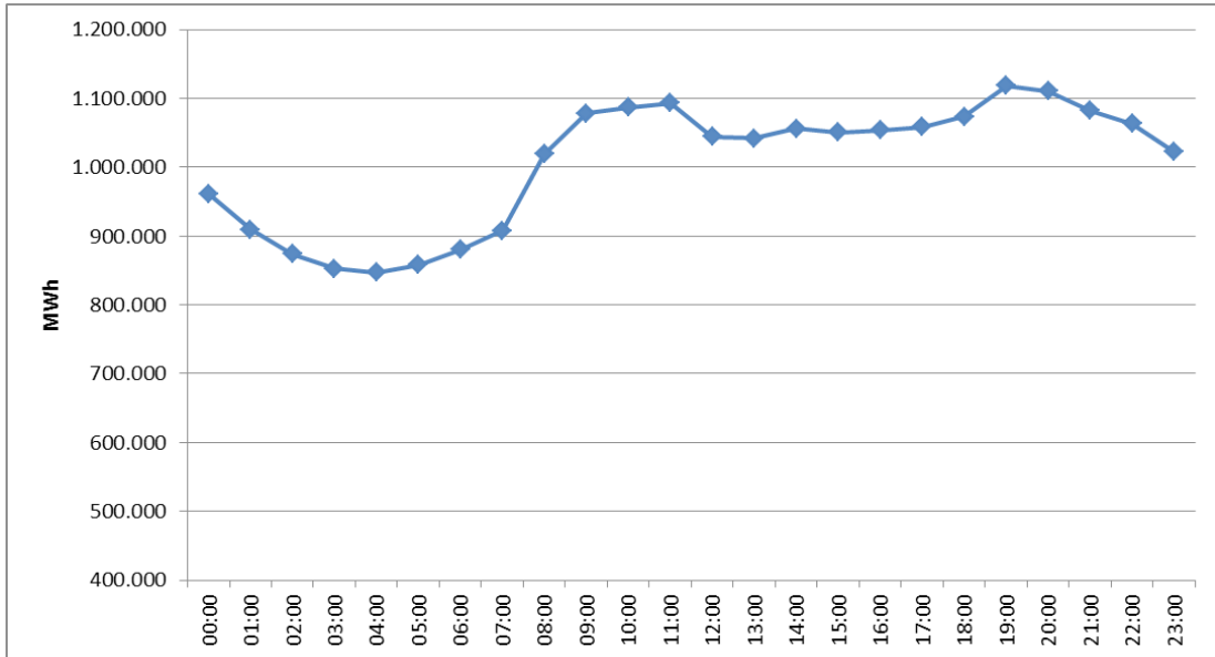
Şekil 2.2. Mart 2018 Döneminde Elektrik Tüketiminin Saat Bazında Dağılımı (MWh)
