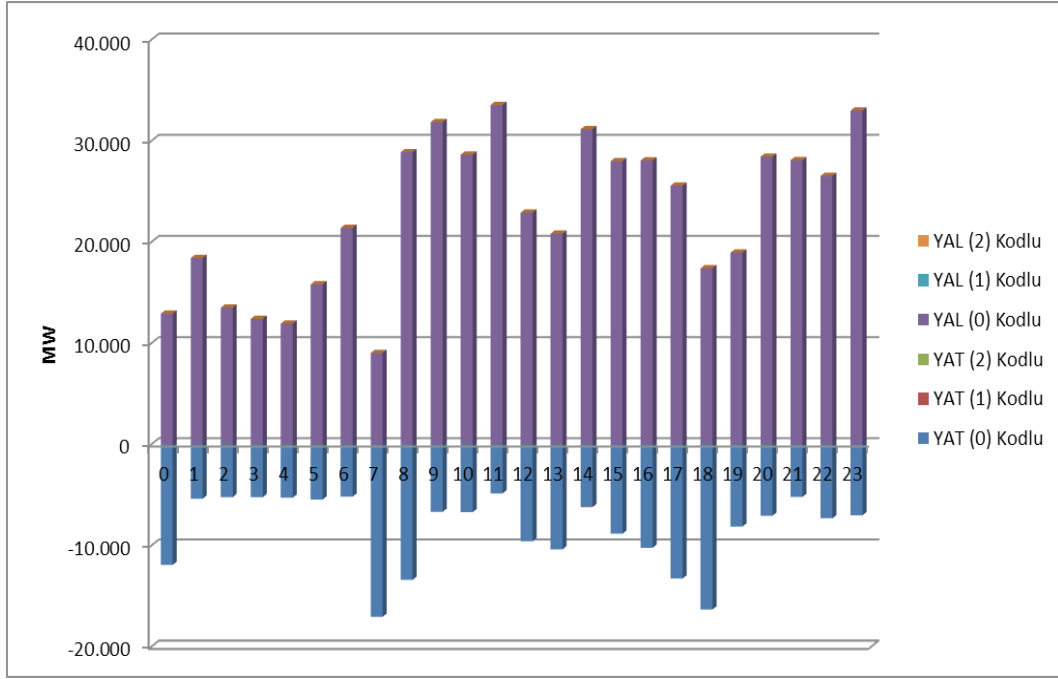
Şekil 4.7 Mart 2018 Döneminde Dengeleme Güç Piyasasında (DGP) Verilen Talimatların Saatlik Bazda Dağılımı (MW)
