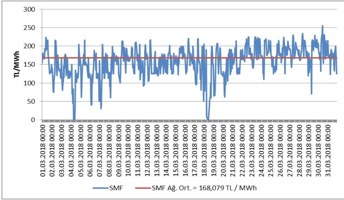
Şekil 4.1 Mart 2018 Döneminde Piyasa Takas Fiyatının (PTF) Saatlik Gelişimi (TL/MWh)
