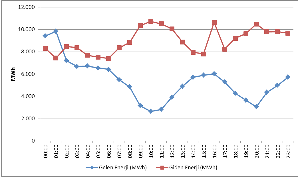
Şekil 3.2. Mart 2018 Döneminde Saatlik Bazda Yurtdışı Elektrik Ticareti (MWh)
