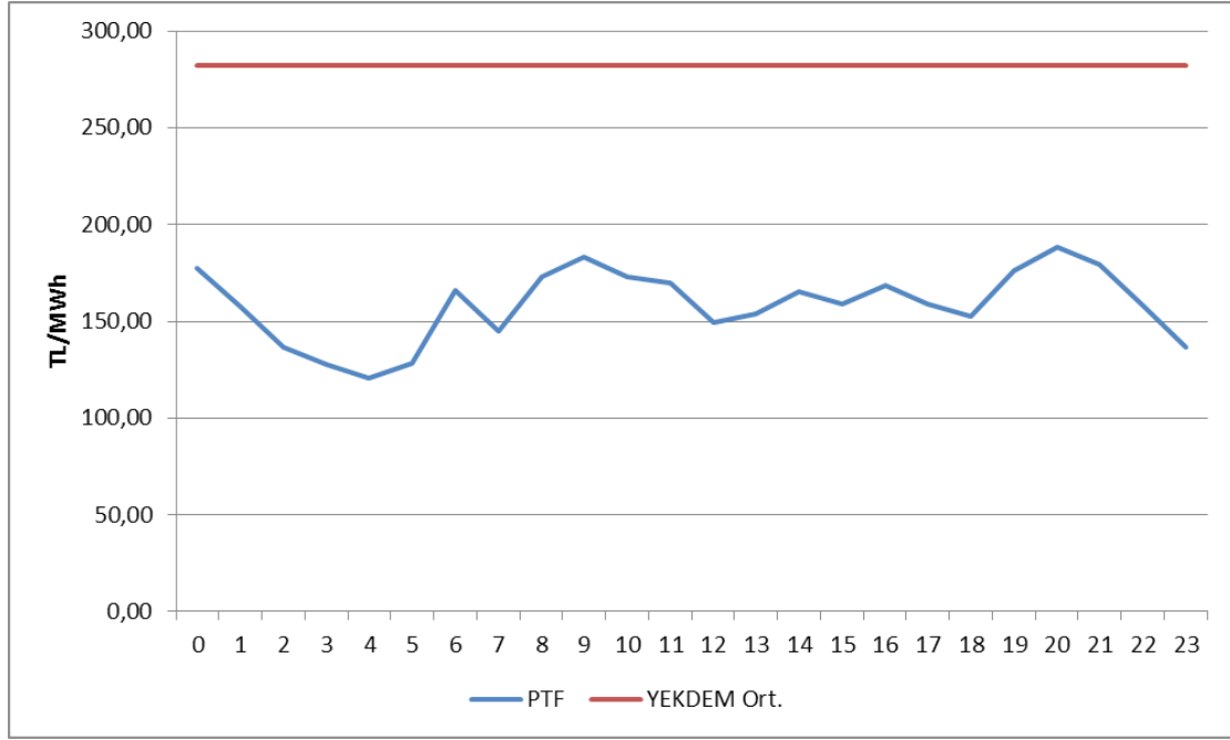
Şekil 1.13 Mart 2018 Döneminde YEKDEM Aylık Ortalama Fiyatı ile Piyasa Takas Fiyatının (PTF) Saatlik Dağılımı (TL/MWh)
