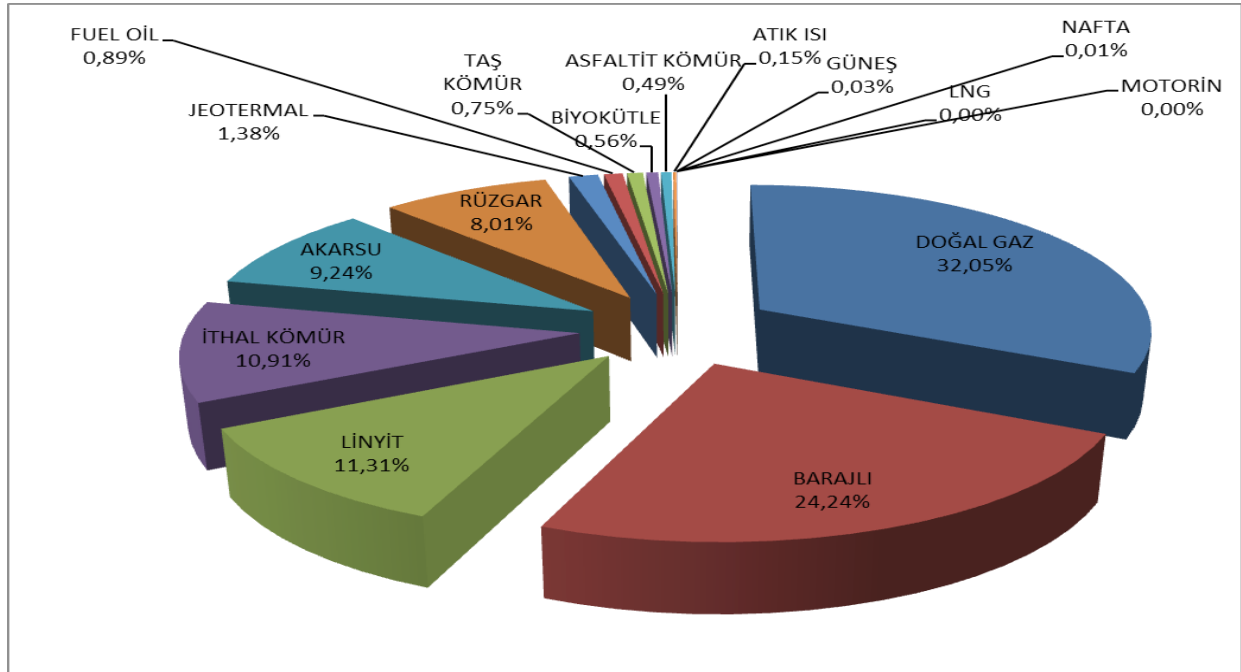
Şekil 1.2 2018 Yılı Mart Ayı Sonu İtibariyle Lisanslı Elektrik Kurulu Gücünün Kaynak Bazında Dağılımı (%)
