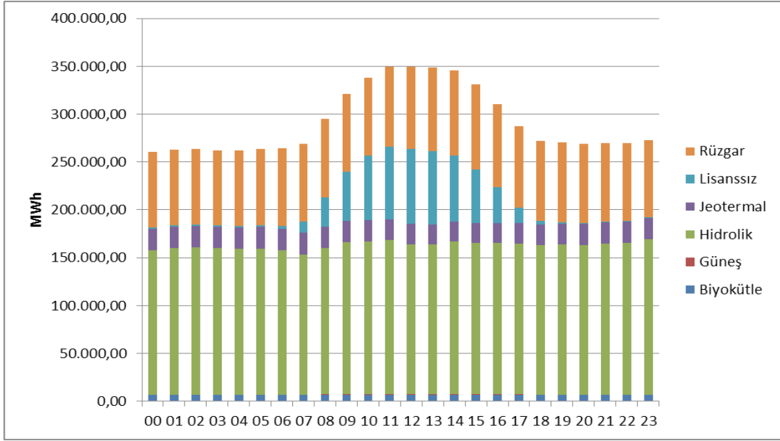
Şekil 1.11 Mart 2018 Döneminde YEKDEM Kapsamındaki Üretimin Saatlik Bazda Kaynaklara Göre Dağılımı (MWh)
