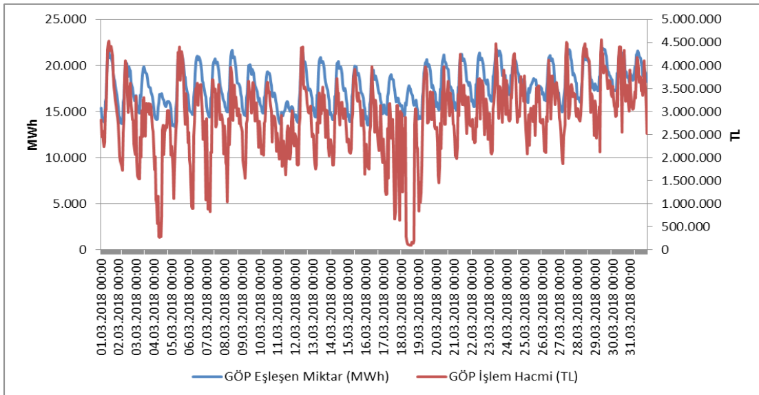
Şekil 4.2 Mart 2018 Döneminde Gün Öncesi Piyasası (GÖP) İşlem Hacminin Saatlik Gelişimi (TL-MWh)
