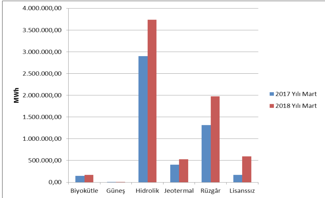
Şekil 1.10 Mart 2018 Döneminde YEKDEM Kapsamındaki Üretim Kaynaklara Göre Dağılımı ve 2017 Yılı Mart Ayı Değeriyle Karşılaştırılması (MWh)
