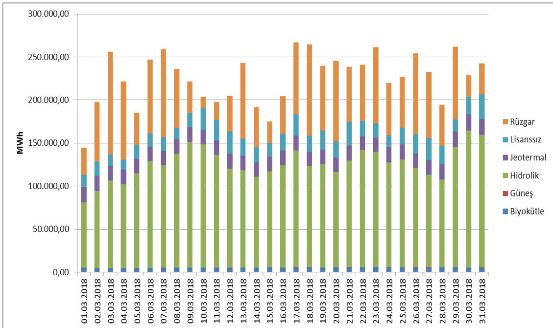
Şekil 1.12 Mart 2018 Döneminde YEKDEM Kapsamındaki Üretimin Günlük Bazda Kaynaklara Göre Dağılımı (MWh)
