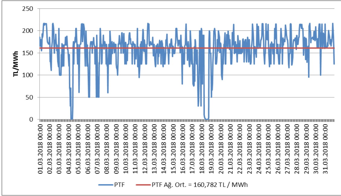
Şekil 4.5 Mart 2018 Döneminde Sistem Marjinal Fiyatının (SMF) Saatlik Gelişimi (TL/MWh)
