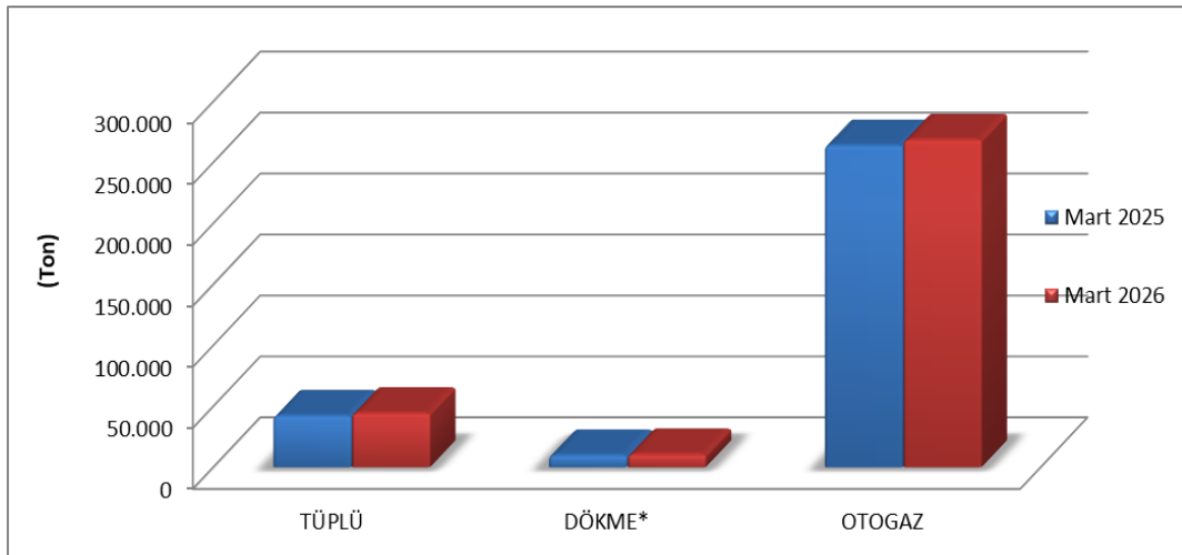
Şekil 3.2: Mart 2025 – Mart 2026 Dönemlerinde Ürün Türüne Göre LPG Satışları
