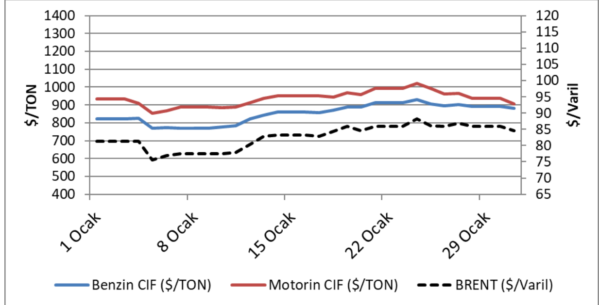
Şekil-1: Ocak Ayı Kurşunsuz Benzin 95 Oktan, Motorin ve Brent (Dated) Seyri-1
