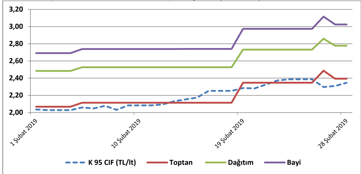
Şekil-3: Kurşunsuz Benzin 95 Oktan Yurt İçi Vergisiz Fiyatının Seyri (TL/lt)
