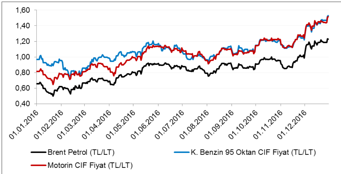
Şekil 7.2. 2016 Yılı Kurşunsuz Benzin 95 Oktan, Motorin ve Brent (Dtd) Seyri
