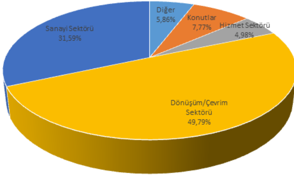
Şekil 5.1 Haziran 2017 Döneminde Sektörel Doğal Gaz Tüketiminin Dağılımı (%)
