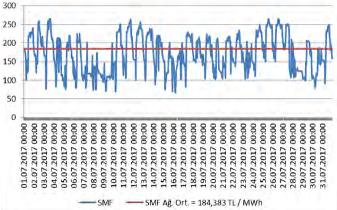
Şekil 4.5 Temmuz 2017 Döneminde Sistem Marjinal Fiyatının (SMF) Saatlik Gelişimi (TL/MWh)
