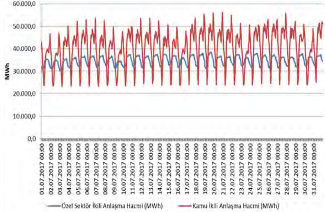
Şekil 4.13 Temmuz 2017 Döneminde İkili Anlaşma Hacminin Saatlik Gelişimi (MWh)
