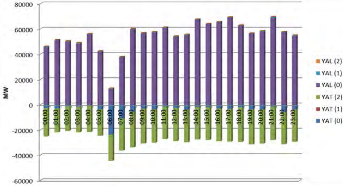
Şekil 4.7 Temmuz 2017 Döneminde Dengeleme Güç Piyasasında (DGP) Verilen Talimatların Saatlik Bazda Dağılımı (MW)
