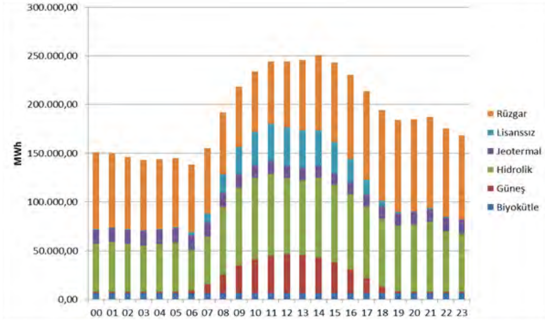
Şekil 1.11 Temmuz 2017 Döneminde YEKDEM Kapsamındaki Üretim Saatlük Bazda Kaynaklara Göre Dağılımı (MWh)
