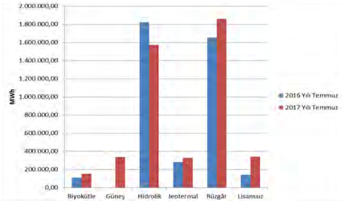
Şekil 1.10 Temmuz 2017 Döneminde YEKDEM Kapsamındaki Üretimin Kaynaklara Göre Dağılımı ve 2016 Yılı Temmuz Ayı Değeriyle Karşılaştırılması (MWh)
