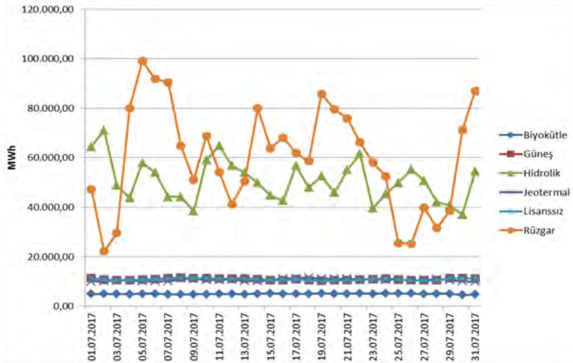
Şekil 1.12 Temmuz 2017 Döneminde YEKDEM Kapsamındaki Üretim Günlük Bazda Kaynaklara Göre Dağılımı (MWh)
