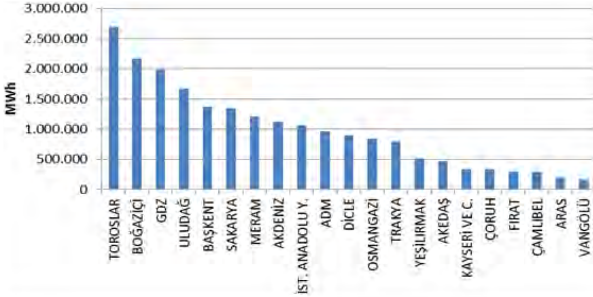
Şekil 2.4 Faturalanan Elektrik Tüketiminin Dağıtım Bölgesi Bazında Dağılımı (MWh)
