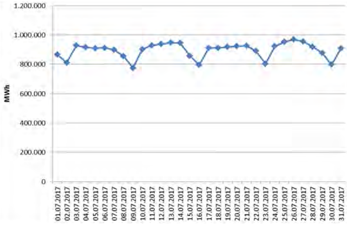
Şekil 2.3. Temmuz 2017 Döneminde Elektrik Tüketiminin Gün Bazında Dağılımı (MWh)
