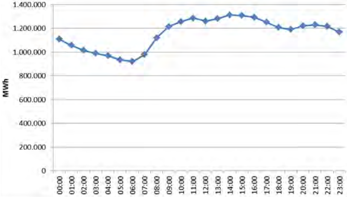
Şekil 2.2. Temmuz 2017 Döneminde Elektrik Tüketiminin Saat Bazında Dağılımı (MWh)
