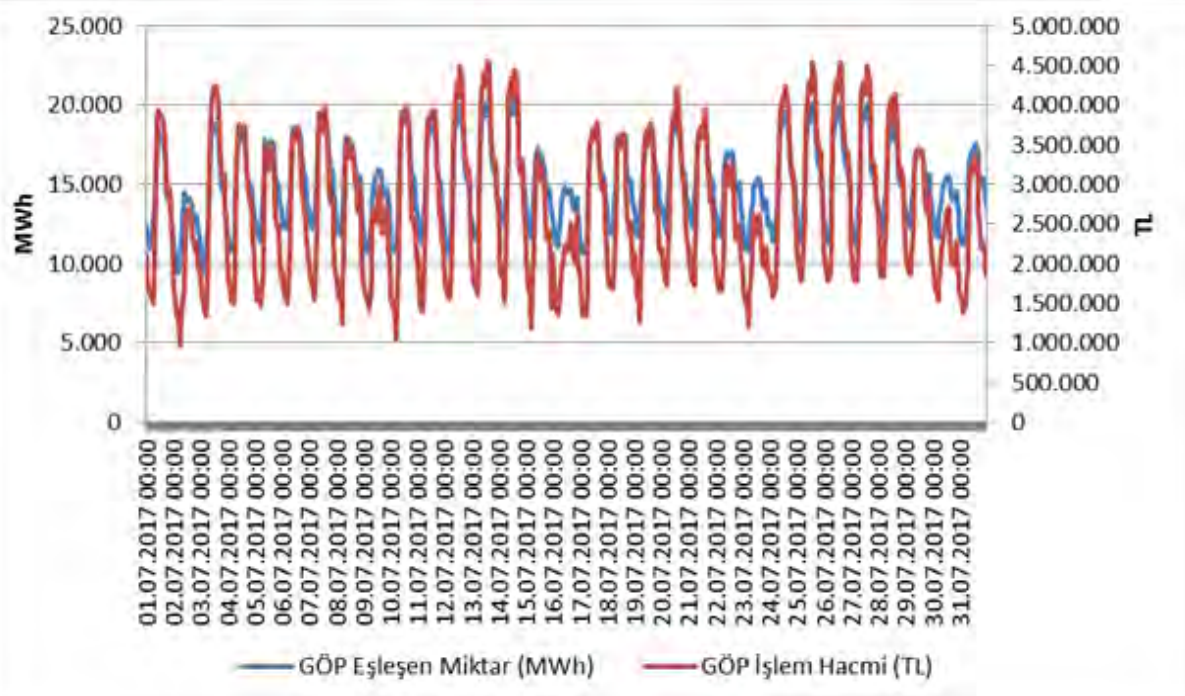
Şekil 4.2 Temmuz 2017 Döneminde Gün Öncesi Piyasası (GÖP) İşlem Hacminin Saatlik Gelişimi (TL-MWh)
