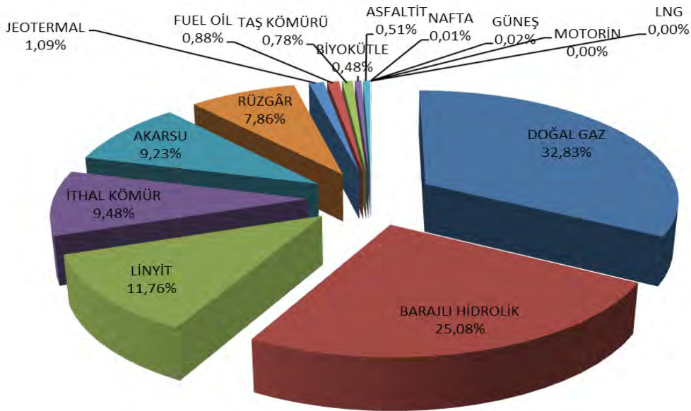
Şekil 1.2 2017 Yılı Temmuz Ayı Sonu İtibariyle Lisanslı Elektrik Kurulu Gücünün Kaynak Bazında Dağılımı (%)
