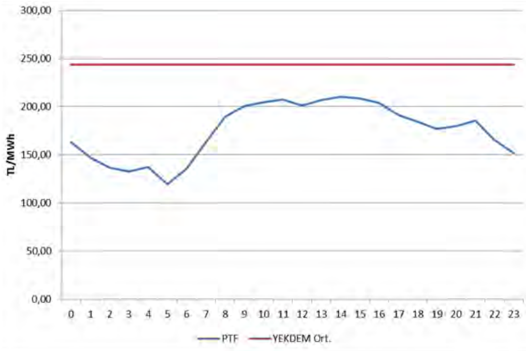
Şekil 1.13 Temmuz 2017 Döneminde YEKDEM Aylık Ortalama Fiyatı ile Piyasa Takas Fiyatının (PTF) Saatlik Dağılımı (TL/MWh)
