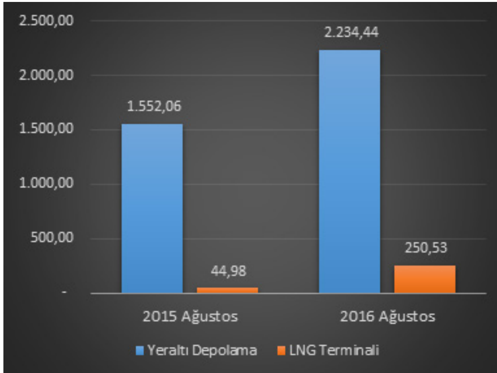
Grafik 3.1 Ağustos 2015 ve Ağustos 2016 Dönemlerindeki Depolama Stok Miktarlarının Depolama Türüne Göre Karşılaştırılması (Milyon Sm 3 )
