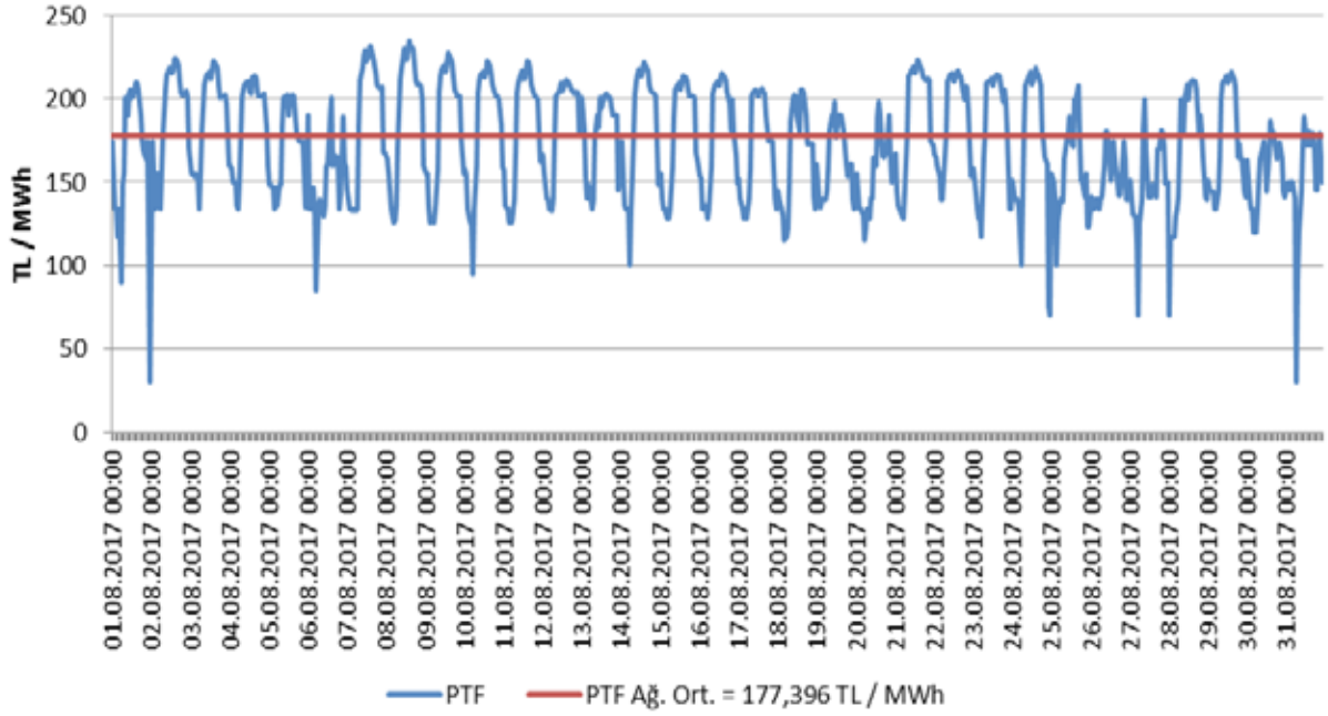
Şekil 4.1 Ağustos 2017 Döneminde Piyasa Takas Fiyatının (PTF) Saatlik Gelişimi (TL/MWh)
