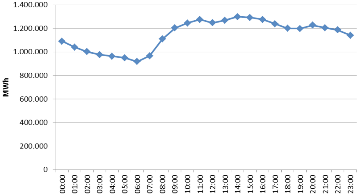
Şekil 2.2. Ağustos 2017 Döneminde Elektrik Tüketiminin Saat Bazında Dağılımı (MWh)
