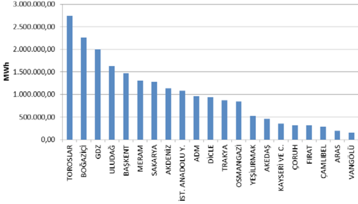
Şekil 2.4 Ağustos 2017 Dönemi Faturalanan Elektrik Tüketiminin Dağıtım Bölgesi Bazında Dağılımı (MWh)
