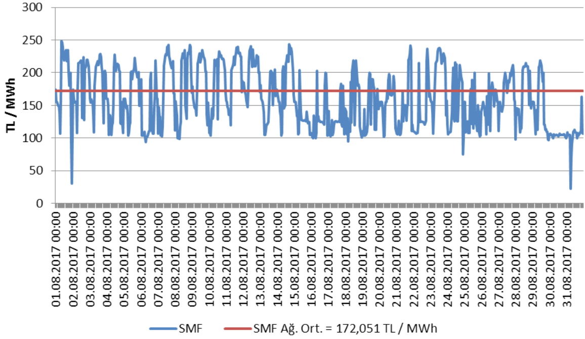
Şekil 4.5 Ağustos 2017 Döneminde Sistem Marjinal Fiyatının (SMF) Saatlik Gelişimi (TL/MWh)
