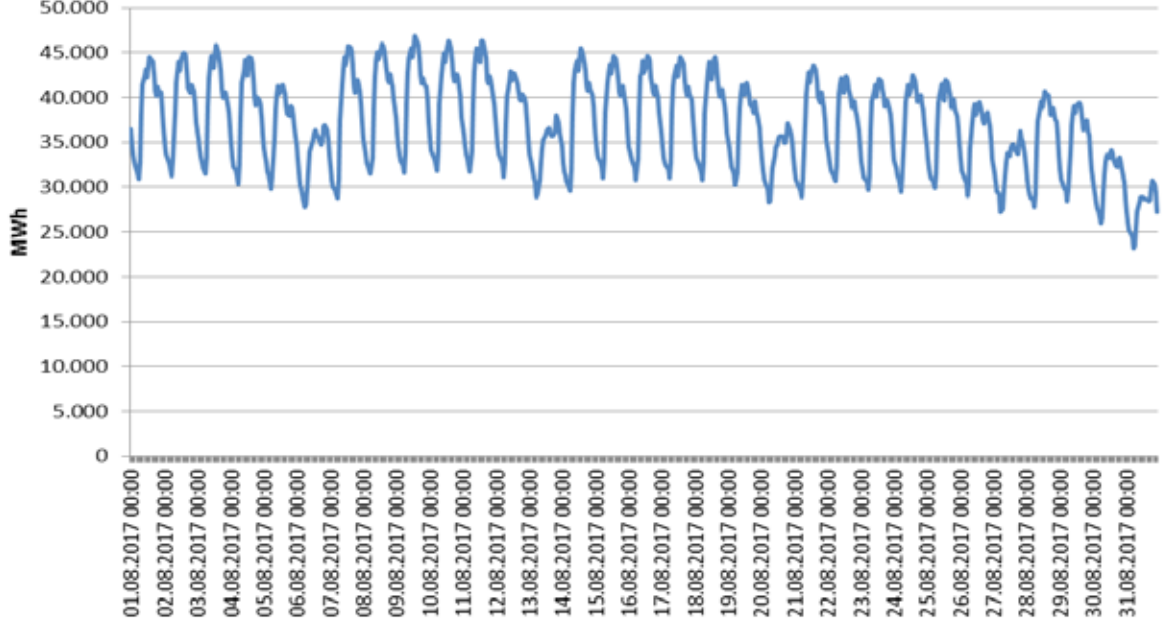
Şekil 2.1. Ağustos 2017 Döneminde Elektrik Tüketiminin Saatlik Gelişimi (MWh)
