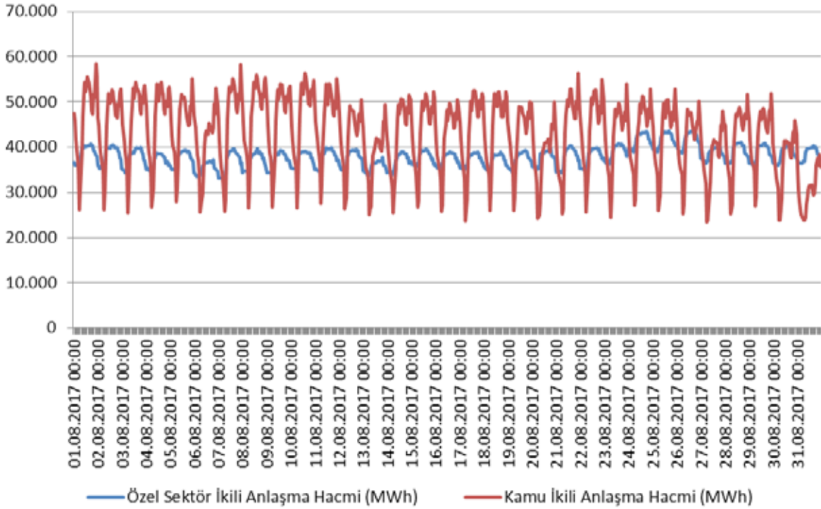
Şekil 4.13 Ağustos 2017 Döneminde İkili Anlaşma Hacminin Saatlik Gelişimi (MWh)
