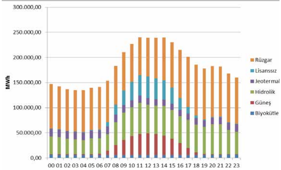
Şekil 1.11 Ağustos 2017 Döneminde YEKDEM Kapsamındaki Üretim Saati Bazda Kaynaklara Göre Dağılımı (MWh)
