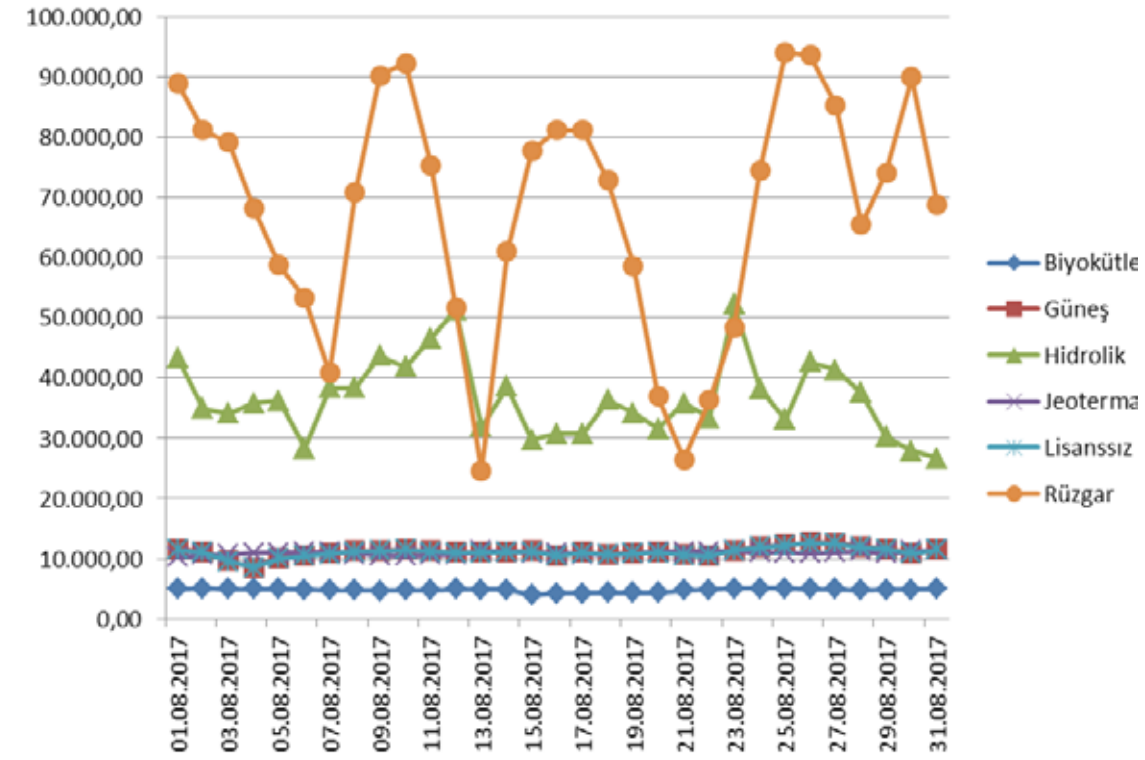
Şekil 1.12 Ağustos 2017 Döneminde YEKDEM Kapsamındaki Üretim Günlük Bazda Kaynaklara Göre Dağılımı (MWh)
