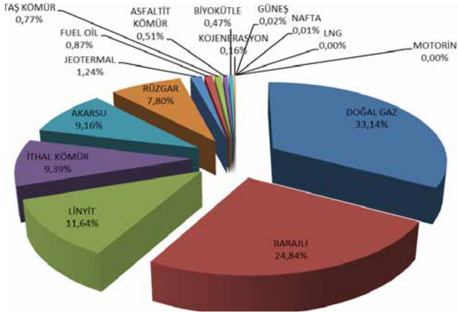
Şekil 1.2 2017 Yılı Ağustos Ayı Sonu İtibariyle Lisanslı Elektrik Kurulu Gücünün Kaynak Bazında Dağılımı (%)
