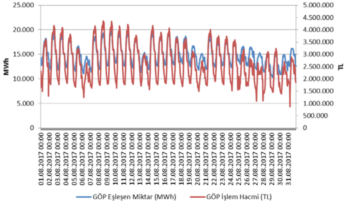
Şekil 4.2 Ağustos 2017 Döneminde Gün Öncesi Piyasası (GÖP) İşlem Hacminin Saatlik Gelişimi (TL-MWh)
