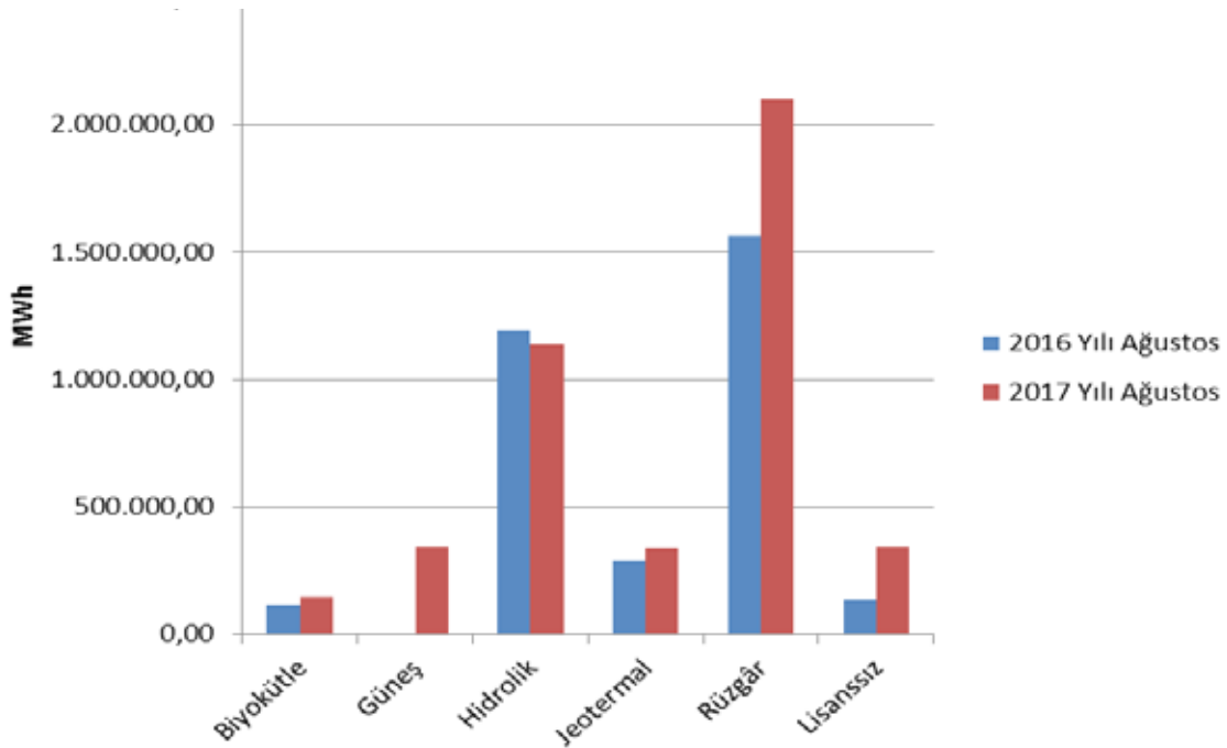
Şekil 1.10 Ağustos 2017 Döneminde YEKDEM Kapsamındaki Üretim Kaynaklara Göre Dağılımı ve 2016 Yılı Ağustos Ayı Değeriyle Karşılaştırılması (MWh)
