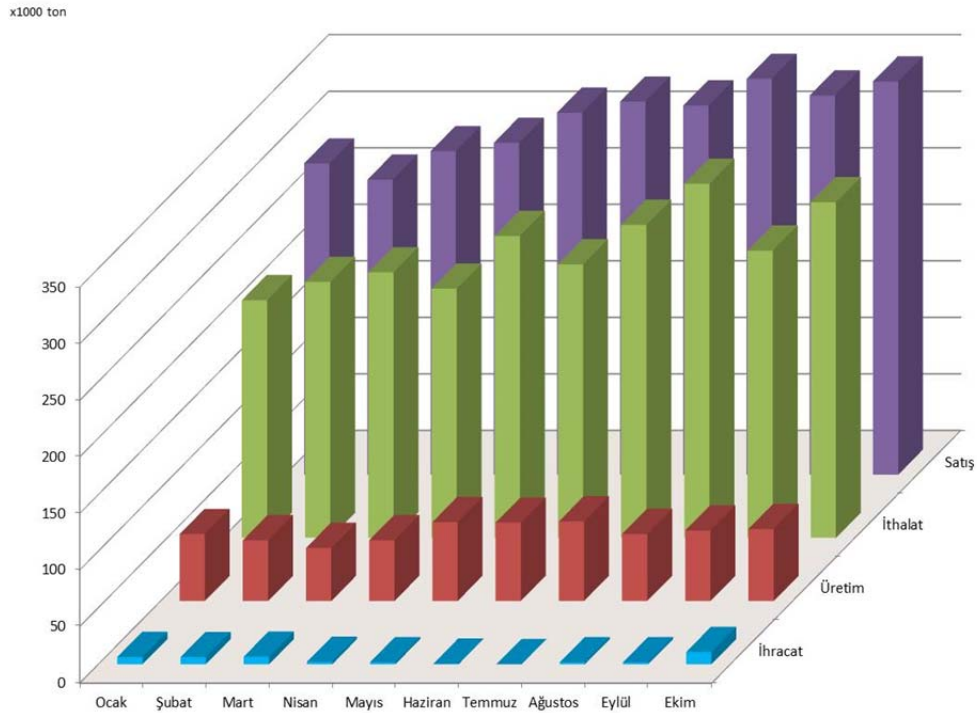
Şekil 4.1.1: Aylık LPG üretim-satış-ithalat-ihracat miktarları
