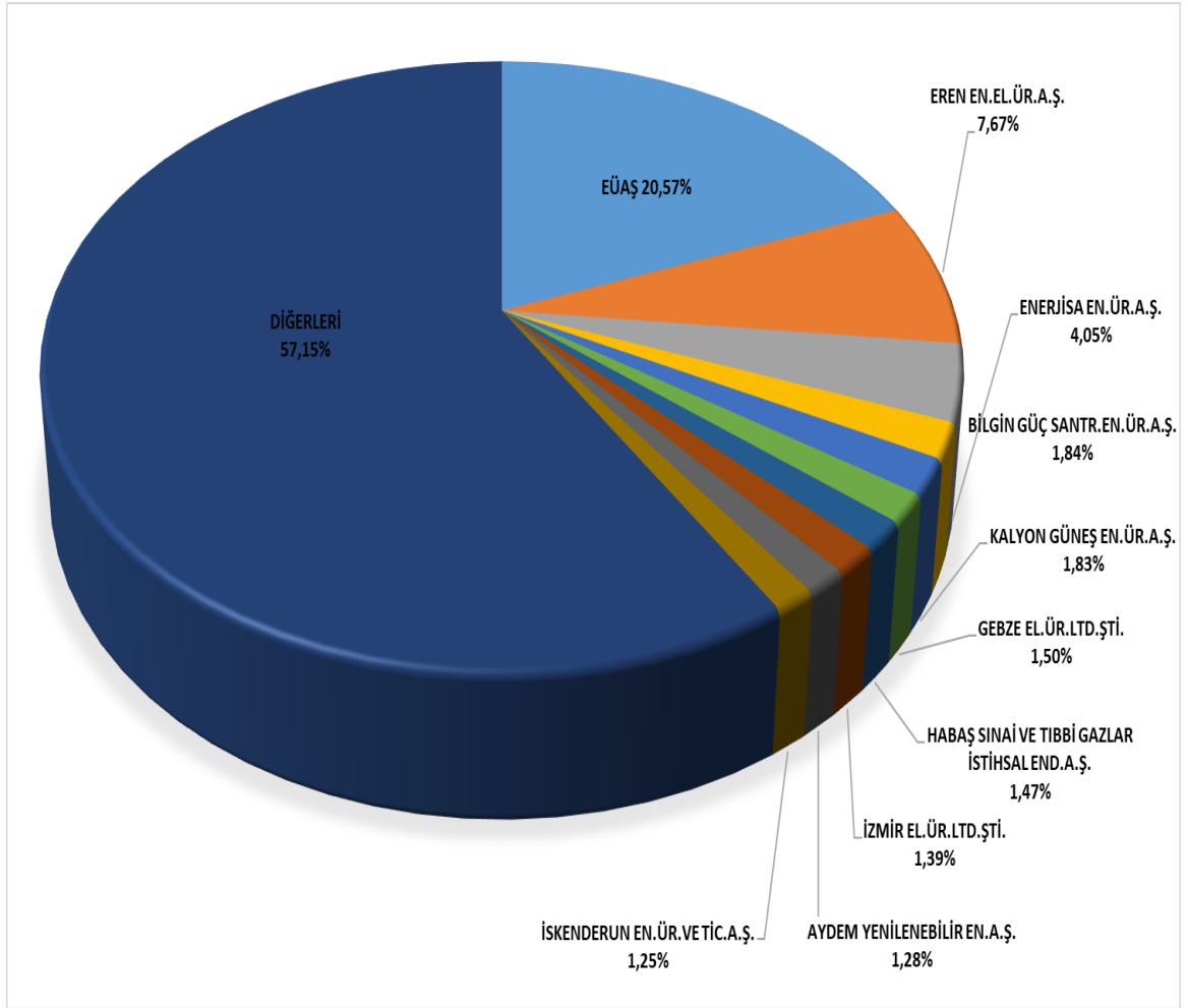
Şekil 1.3 Ağustos 2026 Döneminde Lisanslı Elektrik Kurulu Gücünde İlk 10 Şirketin Payları (%)
