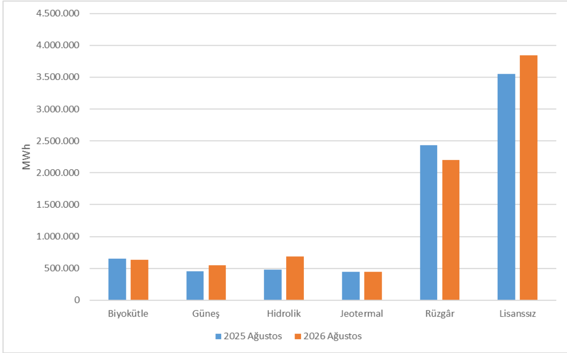
Şekil 1.9 2025-2026 Ağustos Dönemi YEKDEM Kapsamındaki Üretimin Kaynaklara Göre Dağılımı
