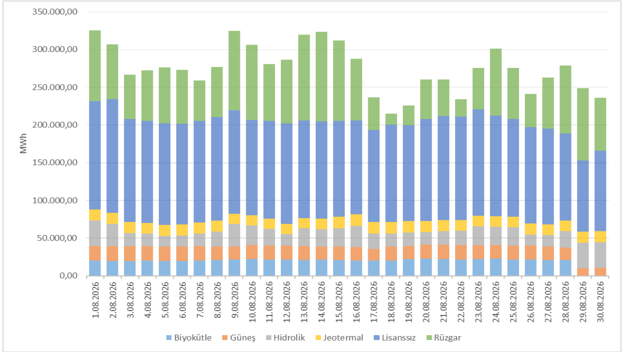
Şekil 1.11 Ağustos 2026 Döneminde YEKDEM Kapsamındaki Üretimin Günlük Bazda Kaynaklara Göre Dağılımı (MWh)
