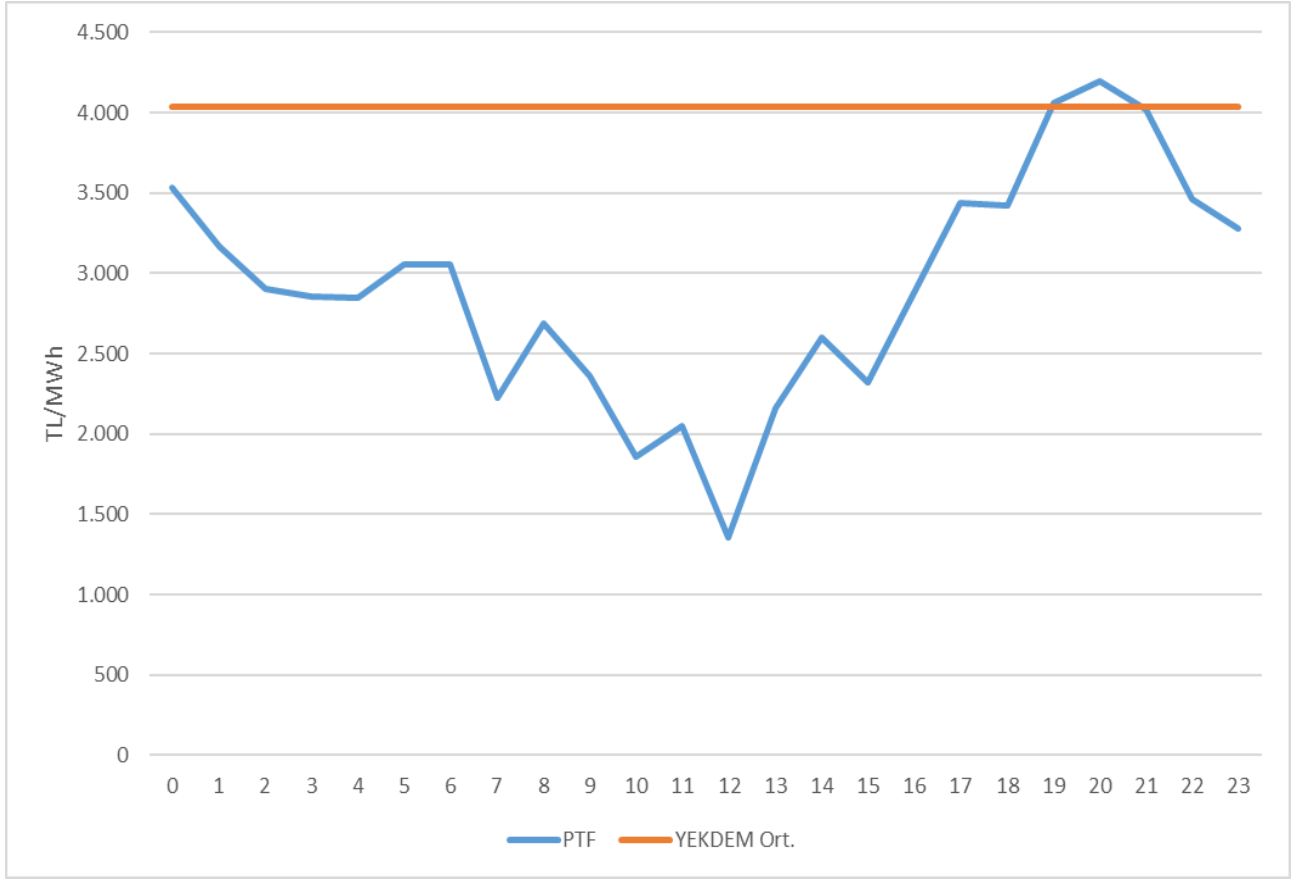
Şekil 1.12 Ağustos 2026 Döneminde YEKDEM Aylık Ortalama Fiyatı ile Piyasa Takas Fiyatının (PTF) Saatlik Dağılımı (TL/MWh)
