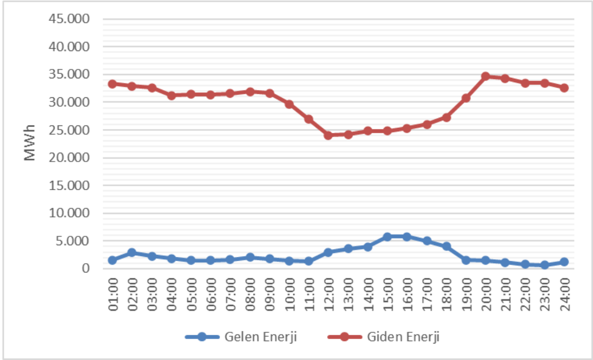
Şekil 3.2 Ağustos 2026 Döneminde Saatlik Bazda Yurtdışı Elektrik Ticareti (MWh)
