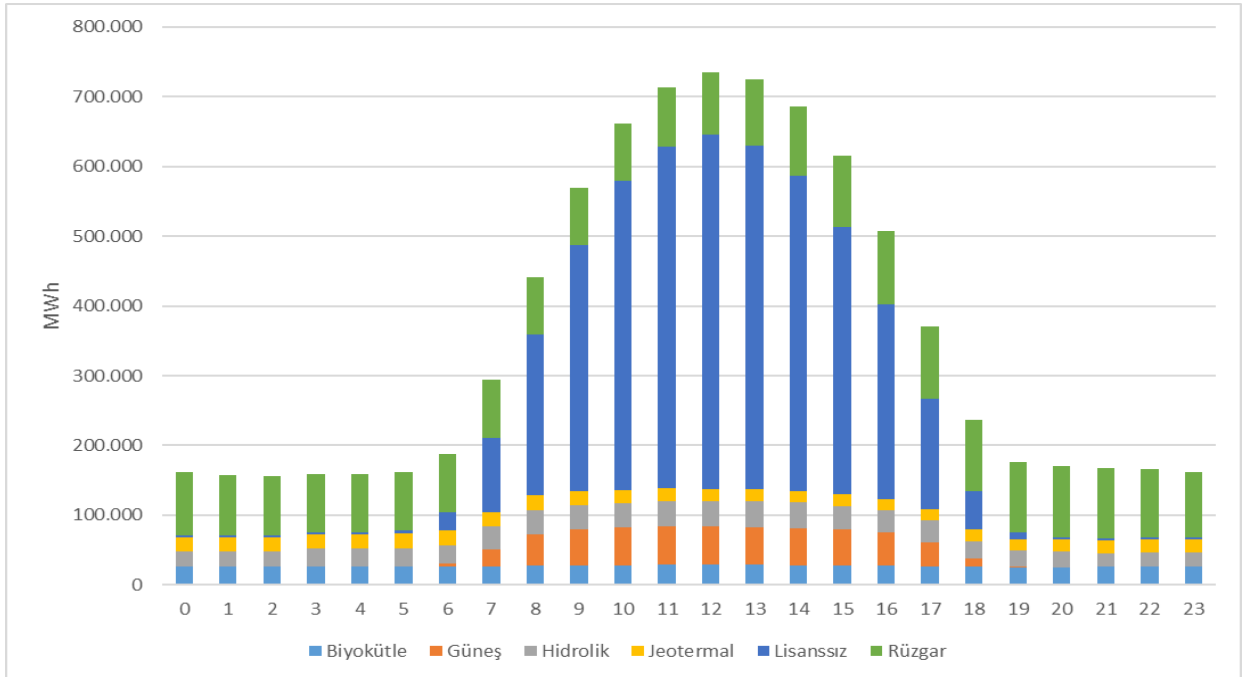
Şekil 1.10 Ağustos 2026 Döneminde YEKDEM Kapsamındaki Üretimin Saatlik Bazda Kaynaklara Göre Dağılımı (MWh)
