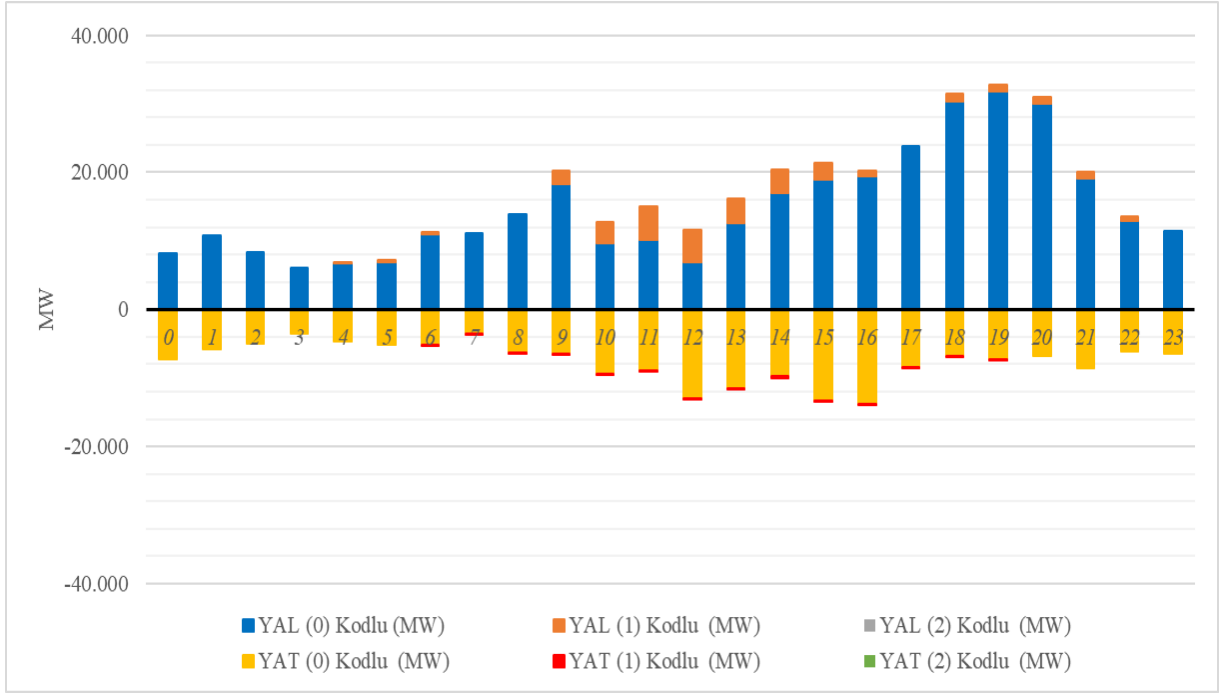
Şekil 4.7 Ağustos 2026 Döneminde Dengeleme Güç Piyasasında (DGP) Verilen Talimatların Saatlik Bazda Dağılımı (MW)
