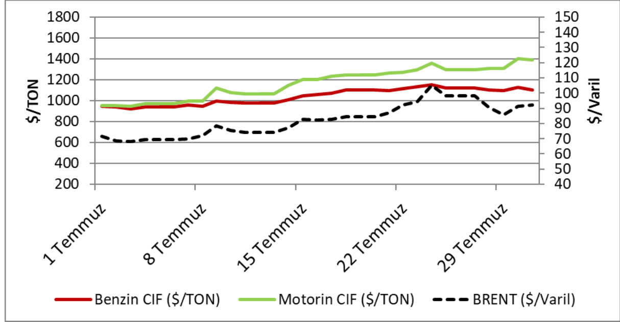
Şekil-1: Temmuz Ayı Kurşunsuz Benzin 95 Oktan, Motorin ve Brent (Dated) Seyri-1
