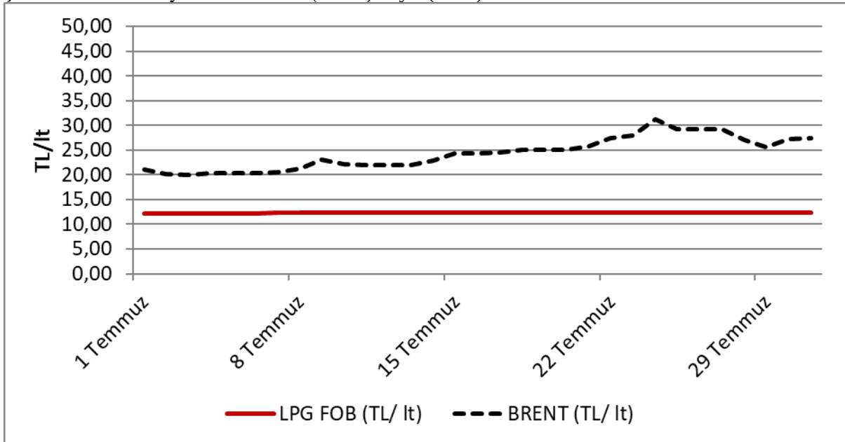
Şekil-8: Temmuz Ayı LPG ve Brent (Dated) Seyri (TL/lt)
