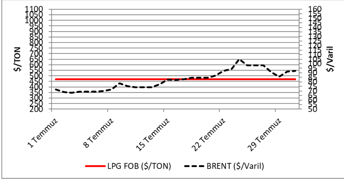
Şekil-7: Temmuz Ayı LPG ($/Ton) ve Brent (Dated-$/Varil) Fiyat Seyri
