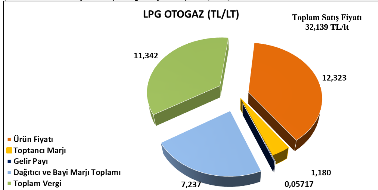
Şekil-9: Temmuz Ayı Yurt İçi Otogaz Fiyat Oluşumu (TL/lt)
