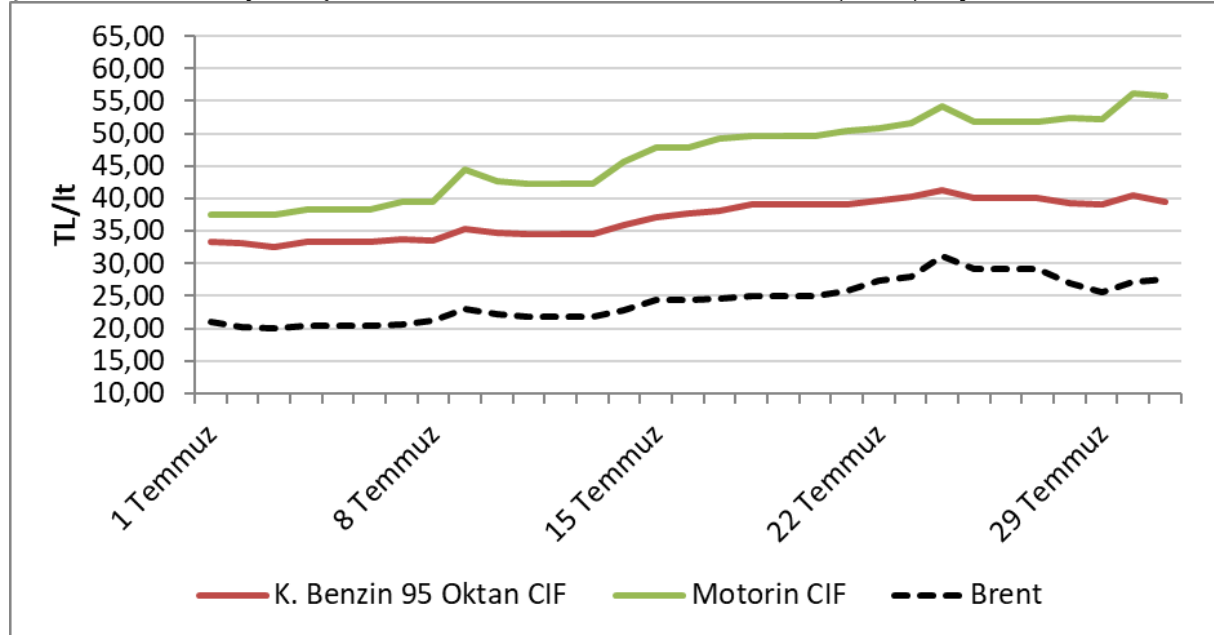
Şekil-2: Temmuz Ayı Kurşunsuz Benzin 95 Oktan, Motorin ve Brent (Dated) Seyri-2
