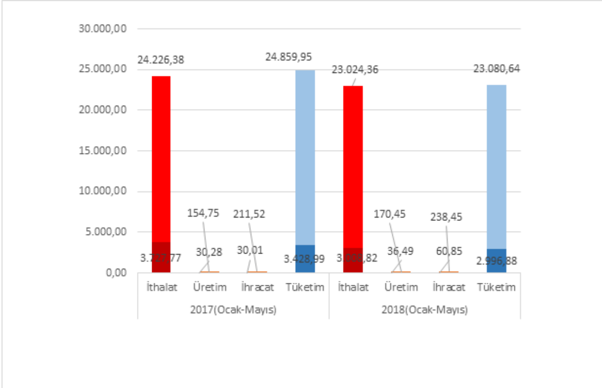
Şekil 1- 2017(Ocak-Mayıs) ve 2018 (Ocak-Mayıs) dönemlerindeki İthalat-Üretim-Tüketim Miktarları ile Mayıs Aylarındaki miktarların bu değerler içerisindeki paylarının Karşılaştırması (Milyon Sm 3 )
