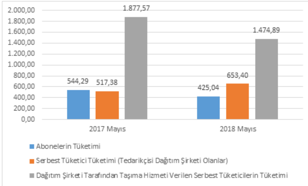
Şekil 5.4 Mayıs 2018 Döneminde Doğal Gaz Dağıtım Bölgelerindeki Toplam Boru Gazı Tüketim Miktarı (Milyon Sm 3 )
