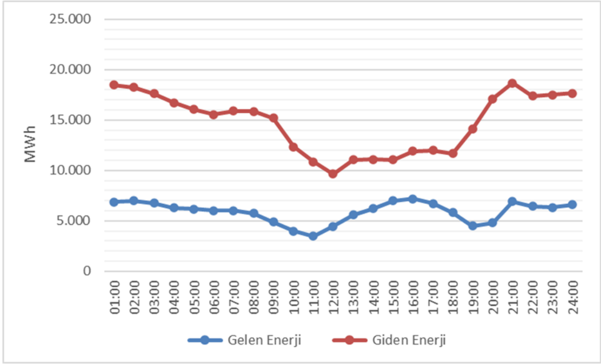
Şekil 3.2 Mayıs 2026 Döneminde Saatlik Bazda Yurtdışı Elektrik Ticareti (MWh)
