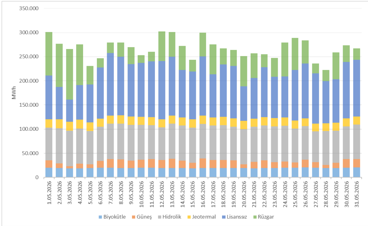
Şekil 1.11 Mayıs 2026 Döneminde YEKDEM Kapsamındaki Üretimin Günlük Bazda Kaynaklara Göre Dağılımı (MWh)
