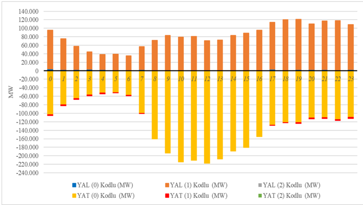
Şekil 4.7 Mayıs 2026 Döneminde Dengeleme Güç Piyasasında (DGP) Verilen Talimatların Saatlik Bazda Dağılımı (MW)
