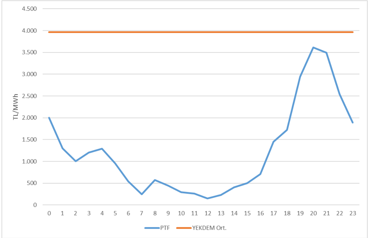
Şekil 1.12 Haziran 2026 Döneminde YEKDEM Aylık Ortalama Fiyatı ile Piyasa Takas Fiyatının (PTF) Saatlik Dağılımı (TL/MWh)
