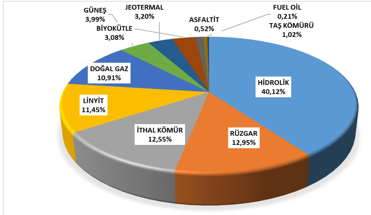
Şekil 1.5 Haziran 2026 Döneminde Lisanslı Elektrik Üretimine Kaynak Bazında Dağılımı (%)
