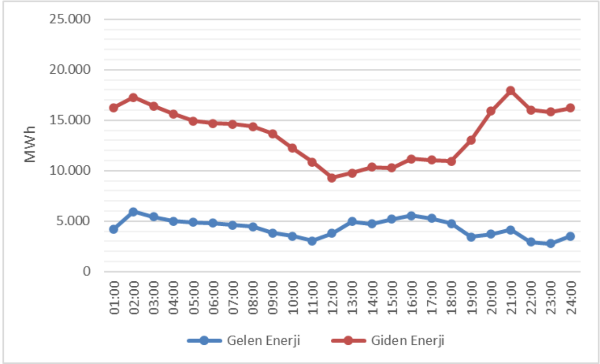
Şekil 3.2 Haziran 2026 Döneminde Saatlik Bazda Yurtdışı Elektrik Ticareti (MWh)
