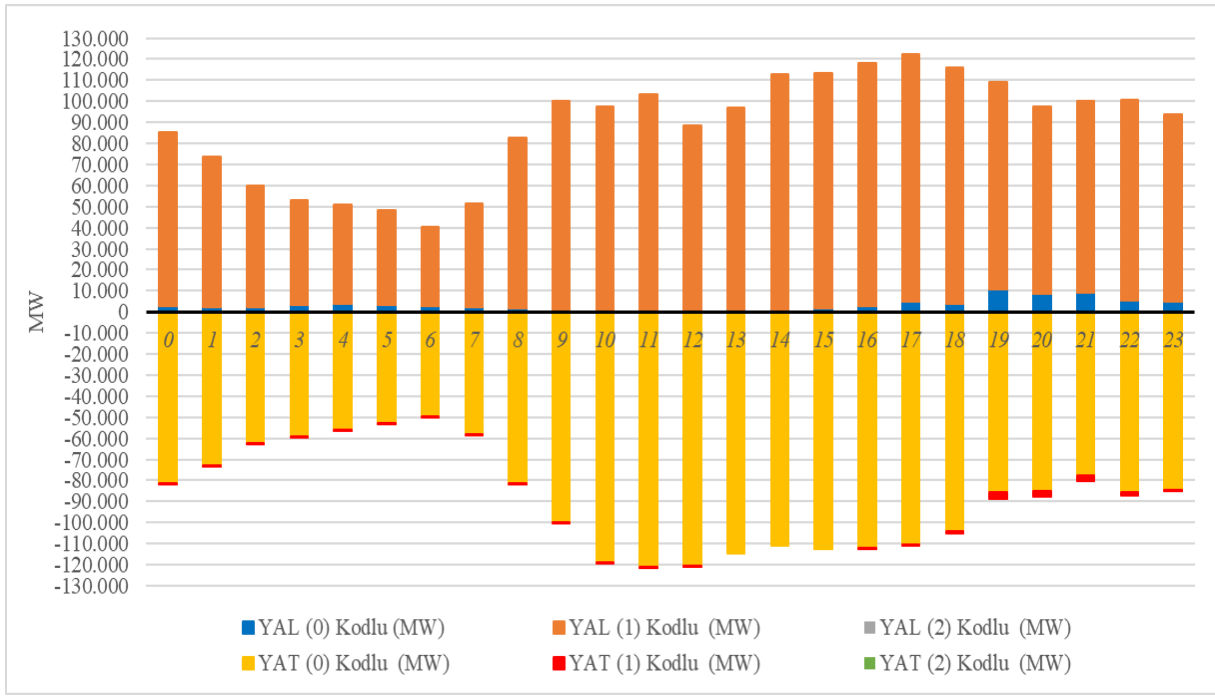
Şekil 4.7 Haziran 2026 Döneminde Dengeleme Güç Piyasasında (DGP) Verilen Talimatların Saatlik Bazda Dağılımı (MW)
