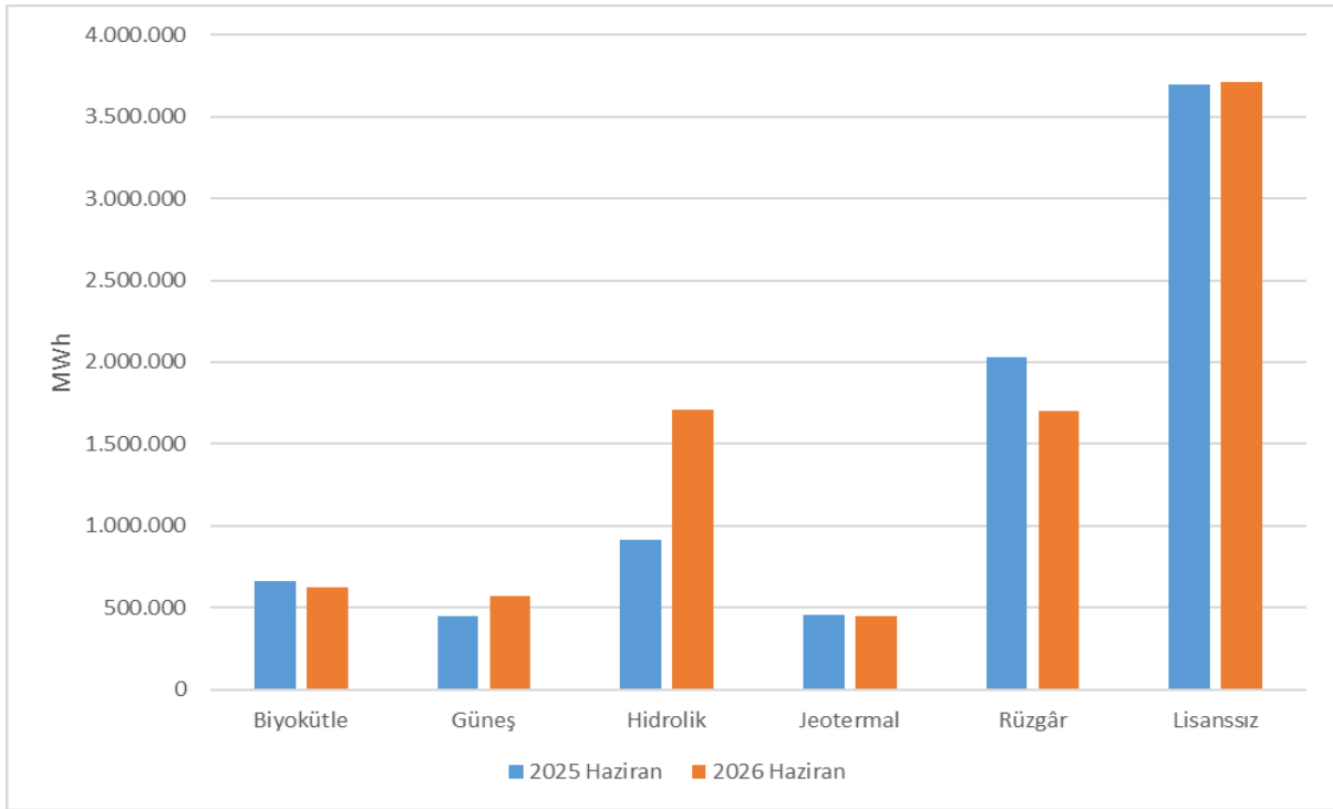
Şekil 1.9 2025-2026 Haziran Dönemi YEKDEM Kapsamındaki Üretimin Kaynaklara Göre Dağılımı
