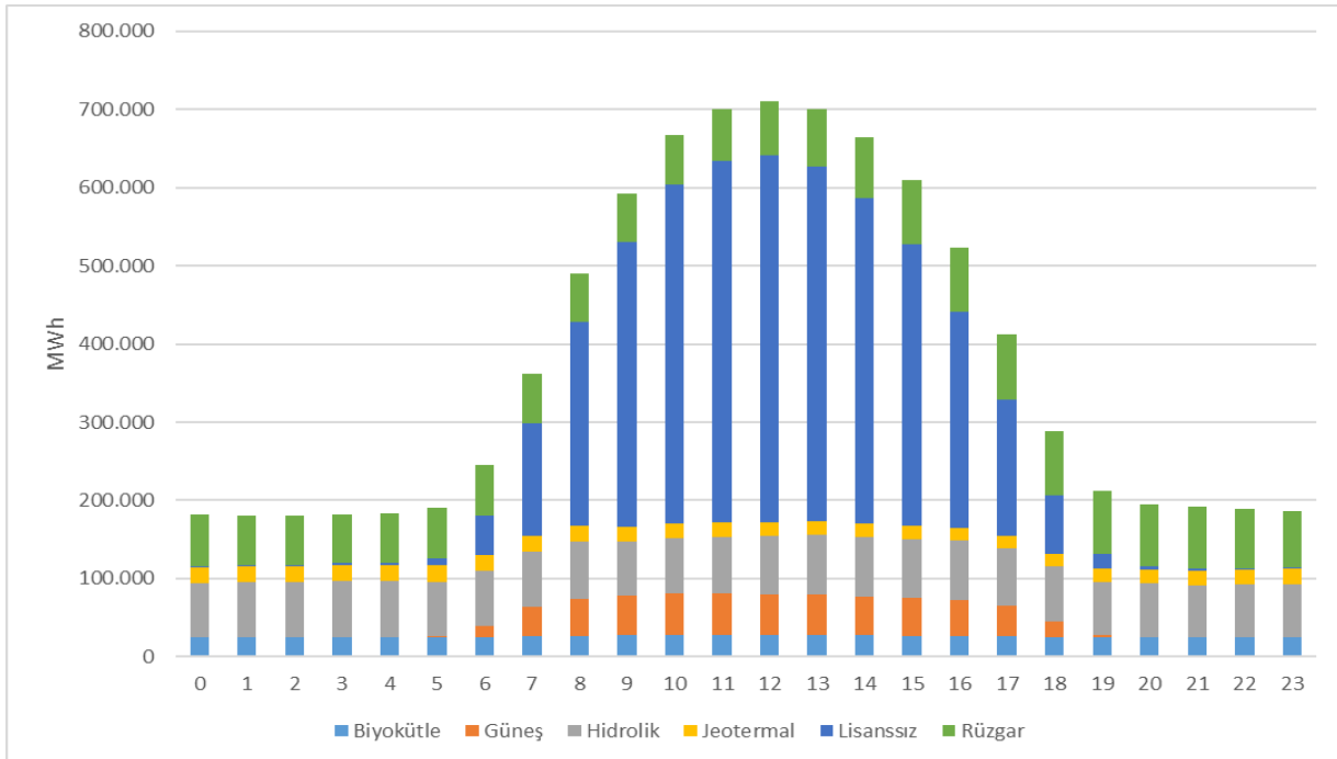
Şekil 1.10 Haziran 2026 Döneminde YEKDEM Kapsamındaki Üretimin Saatlik Bazda Kaynaklara Göre Dağılımı (MWh)
