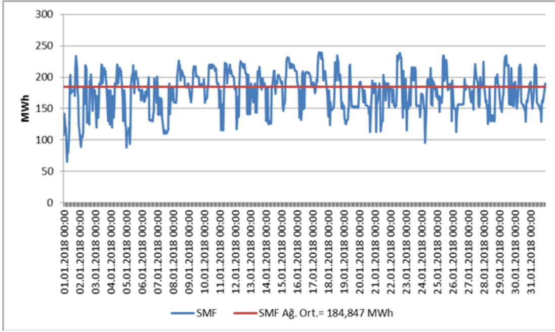
Şekil 4.5 Ocak 2018 Döneminde Sistem Marjinal Fiyatının (SMF) Saatlik Gelişimi (TL/MWh)
