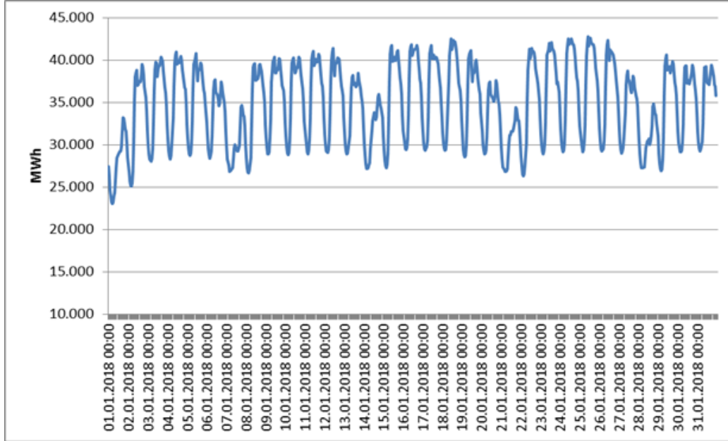
Şekil 2.1. Ocak 2018 Döneminde Elektrik Tüketiminin Saatlik Gelişimi (MWh)
