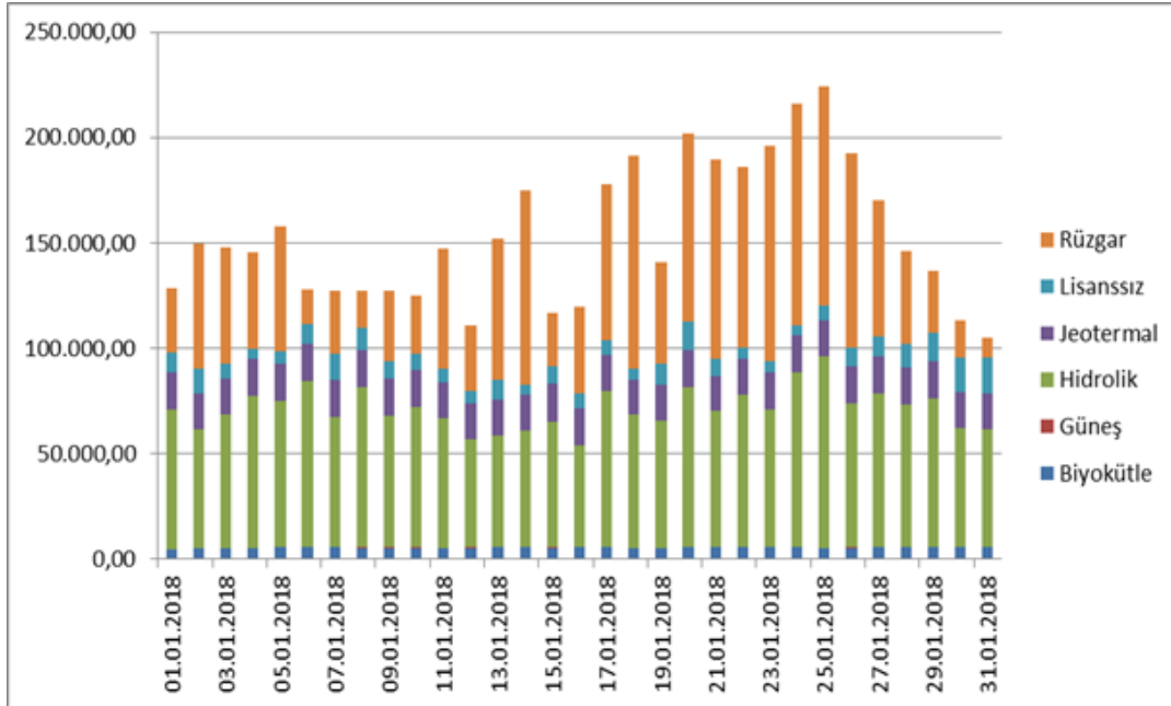
Şekil 1.12 Ocak 2018 Döneminde YEKDEM Kapsamındaki Üretim Günlük Bazda Kaynaklara Göre Dağılımı (MWh)
