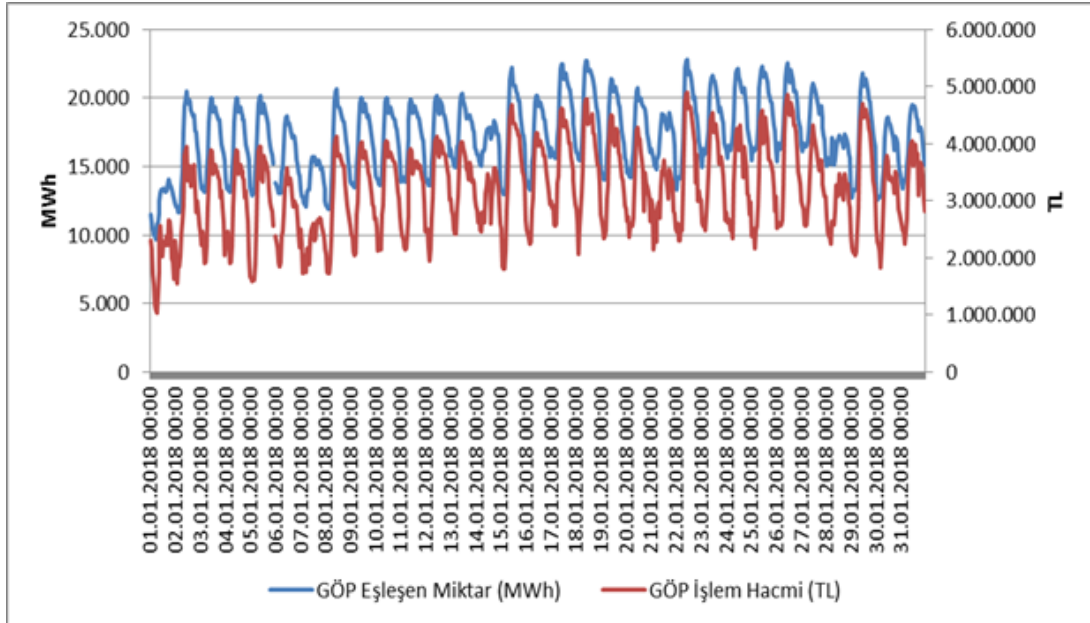
Şekil 4.2 Ocak 2018 Döneminde Gün Öncesi Piyasası (GÖP) İşlem Hacminin Saatlik Gelişimi (TL-MWh)
