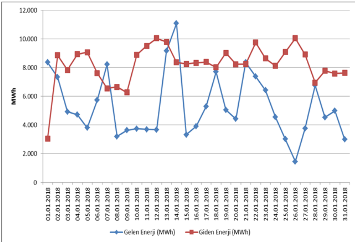
Şekil 3.1. Ocak 2018 Döneminde Günlük Bazda Yurtdışı Elektrik Ticareti (MWh)
