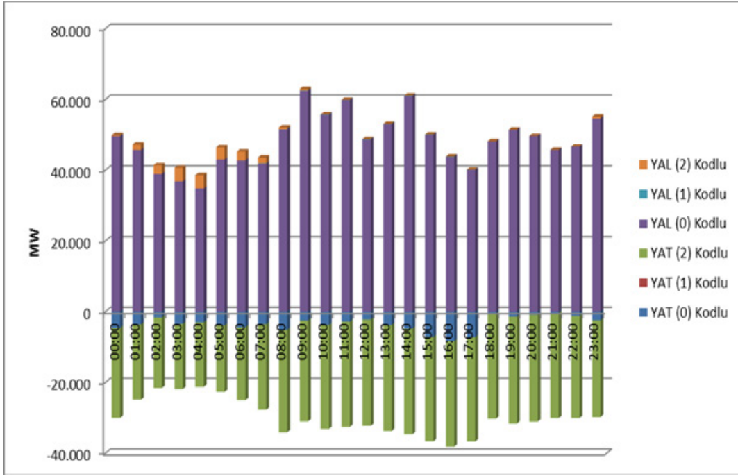
Şekil 4.7 Ocak 2018 Döneminde Dengeleme Güç Piyasasında (DGP) Verilen Talimatların Saatlik Bazda Dağılımı (MW)
