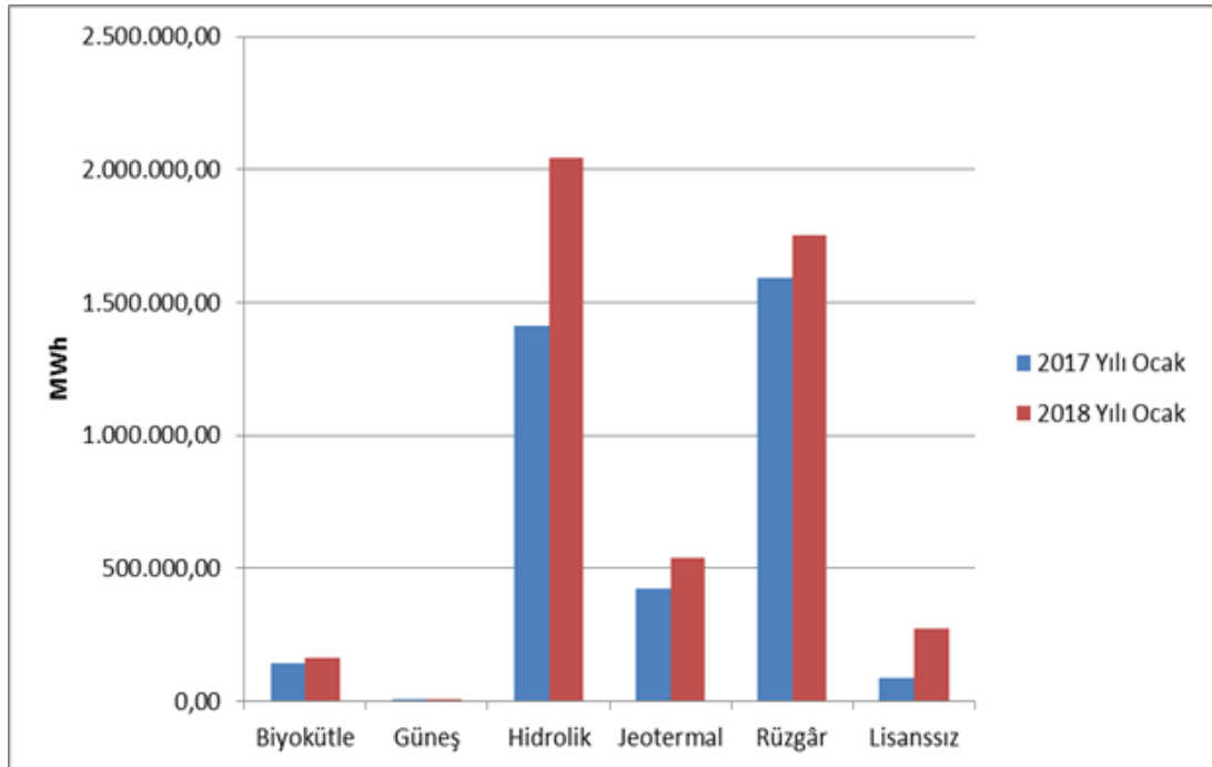
Şekil 1.10 Ocak 2018 Döneminde YEKDEM Kapsamındaki Üretim Kaynaklara Göre Dağılımı ve 2017 Yılı Ocak Ayı Değeriyle Karşılaştırılması (MWh)
