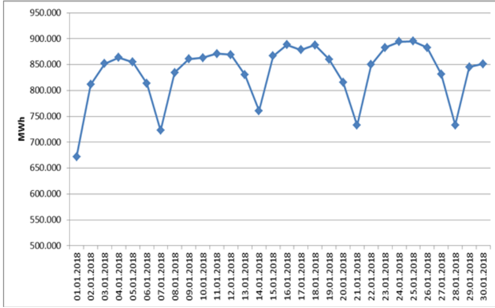
Şekil 2.3. Ocak 2018 Döneminde Elektrik Tüketiminin Gün Bazında Dağılımı (MWh)
