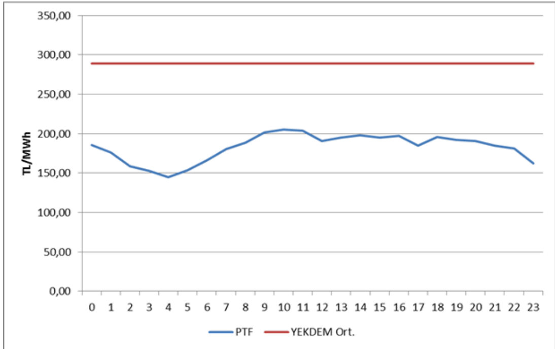
Şekil 1.13 Ocak 2018 Döneminde YEKDEM Aylık Ortalama Fiyatı ile Piyasa Takas Fiyatının (PTF) Saatlik Dağılımı (TL/MWh)
