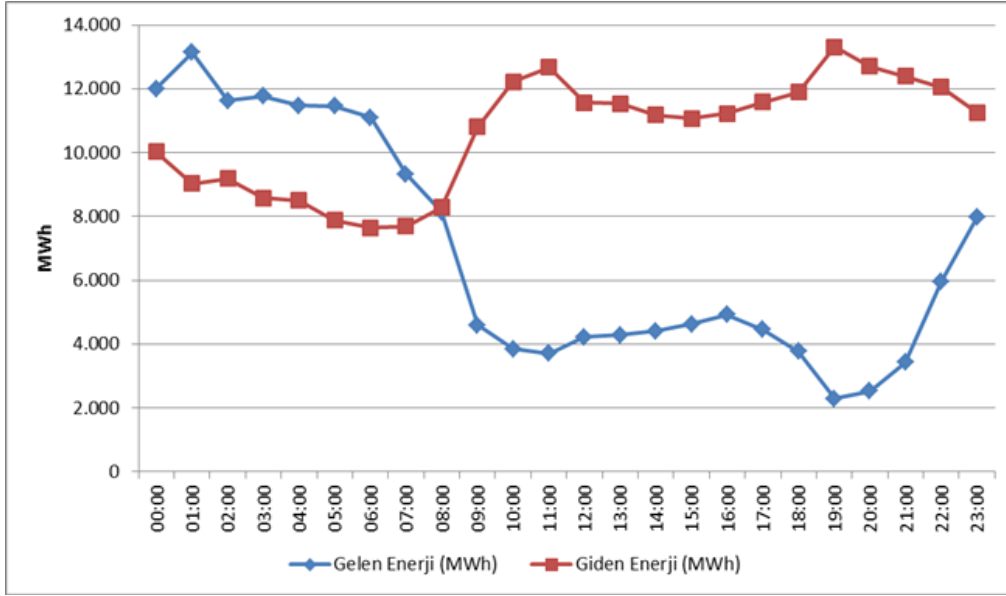
Şekil 3.2. Ocak 2018 Döneminde Saatlik Bazda Yurtdışı Elektrik Ticareti (MWh)
