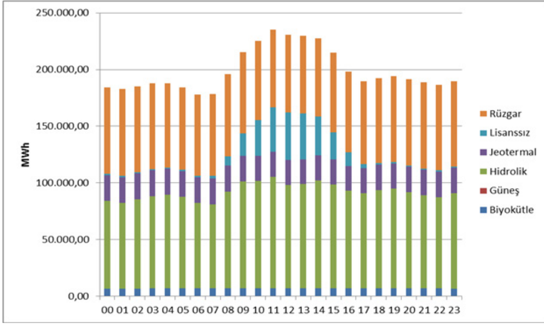
Şekil 1.11 Ocak 2018 Döneminde YEKDEM Kapsamındaki Üretim Saatlik Bazda Kaynaklara Göre Dağılımı (MWh)
