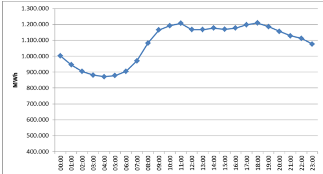
Şekil 2.2. Ocak 2018 Döneminde Elektrik Tüketiminin Saat Bazında Dağılımı (MWh)
