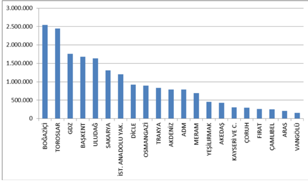
Şekil 2.4 Ocak 2018 Dönemi Faturalanan Elektrik Tüketiminin Dağıtım Bölgesi Bazında Dağılımı (MWh)
