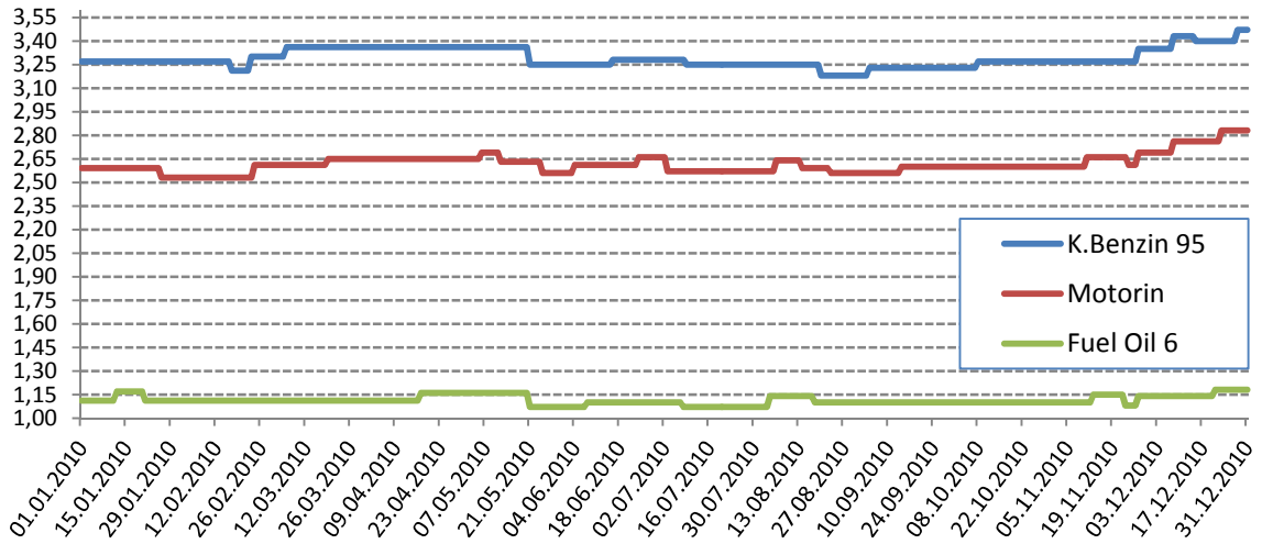
Şekil 4.2 - Toptan Fiyat Değişimi (Vergili)
