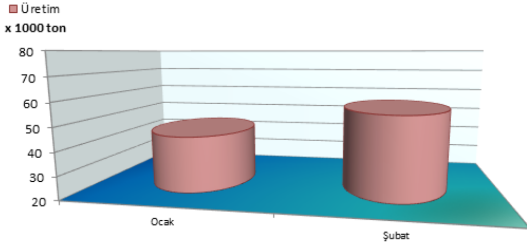
Şekil 3.1.1: Aylık LPG üretim miktarı ve değişimi
