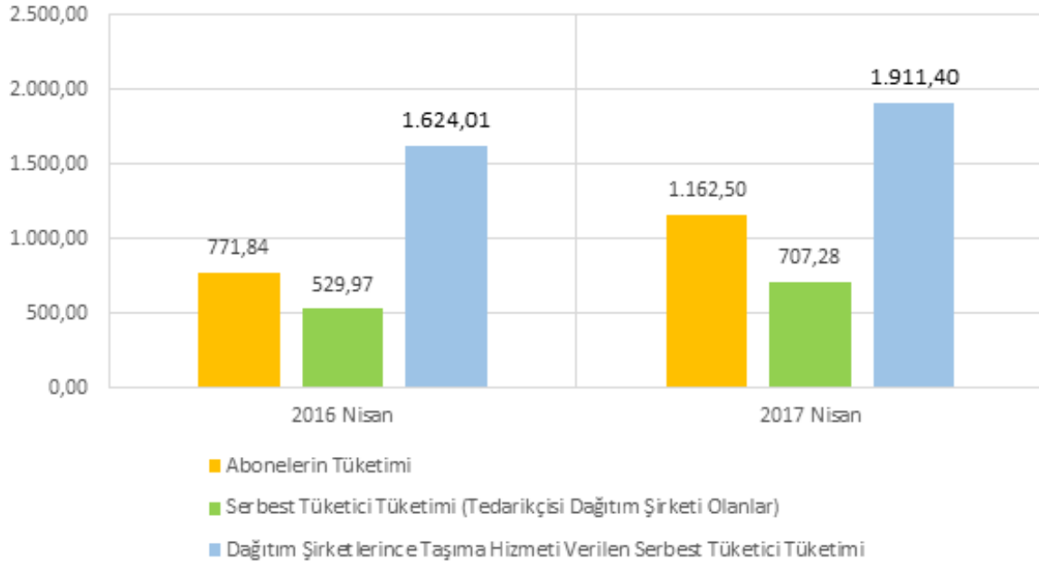
Şekil 5.4 Nisan 2017 Döneminde Doğal Gaz Dağıtım Bölgelerindeki Toplam Boru Gazı Tüketim Miktarı (Milyon Sm 3 )
