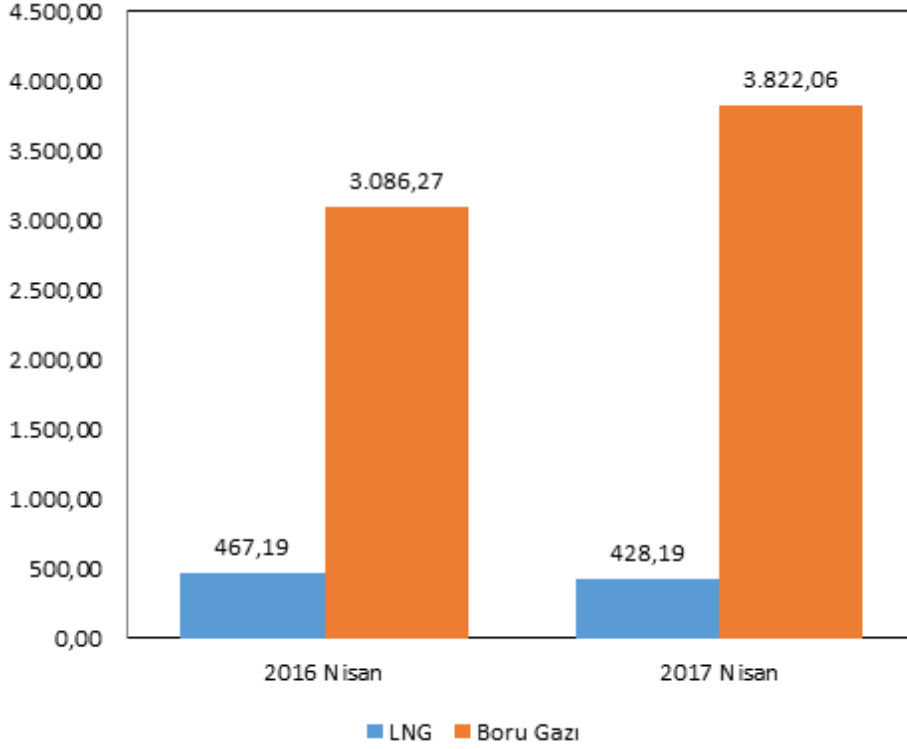
Şekil 2.2 Nisan 2016 ve Nisan 2017 Dönemlerindeki Doğal Gaz İthalat Miktarlarının Gazın Türüne Göre Karşılaştırılması (Milyon Sm 3 )
