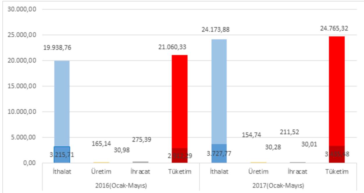
Şekil 1- 2016 (Ocak-Mayıs) ve 2017 (Ocak-Mayıs) dönemlerindeki İthalat-Üretim-Tüketim-Stok Miktarları ile Mayıs Aylarındaki miktarların bu değerler içerisindeki paylarının Karşılaştırması (Milyon Sm 3 )
