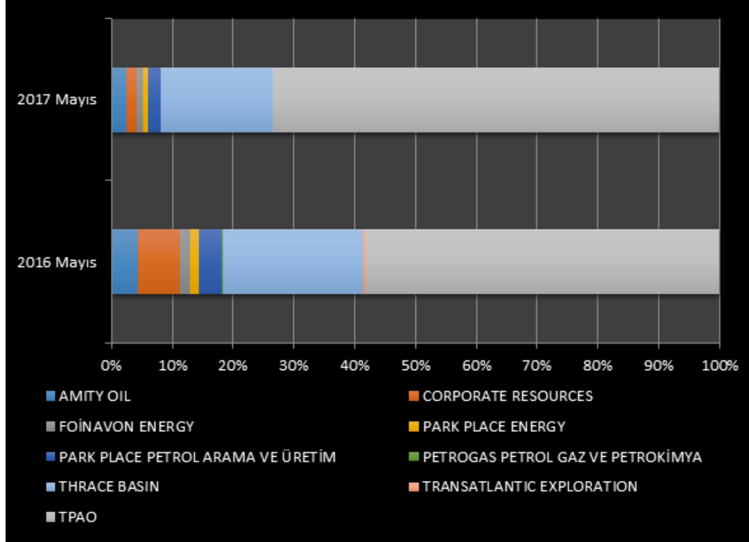
Şekil 1.3 Mayıs 2016 ve Mayıs 2017 Dönemlerinde Toptan Satış Lisansı Sahibi Üretim Şirketlerinin Doğal Gaz Üretim Miktarları Oranlarının Karşılaştırılması (%)
