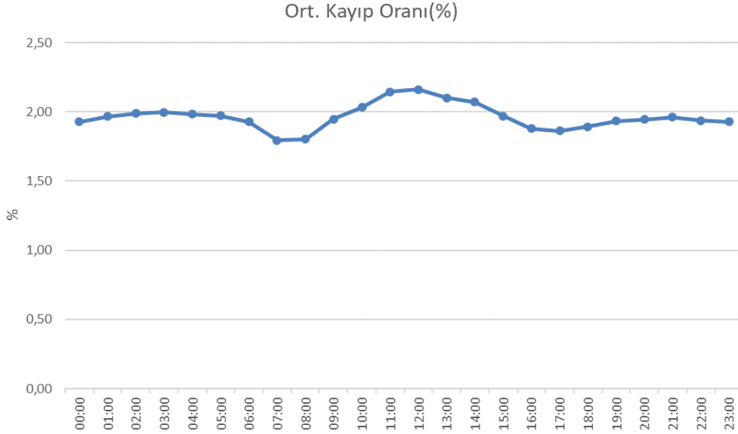
Şekil 4.4: İletim Sistemi Kayıplarının Saatlara Göre Dağılımı (%)
