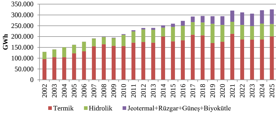
Şekil 1.8: Yıllar İtibarıyla Lisanslı Elektrik Üretiminin Kaynak Bazında Gelişimi (GWh)
