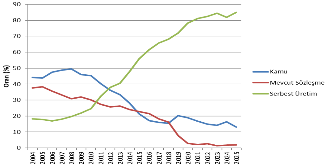
Şekil 1.6: Yıllar İtibarıyla Lisanslı Elektrik Üretiminin Kamu-Özel Olarak Değişimi (%)
