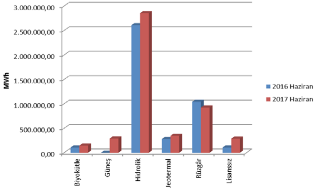
Şekil 1.10 Haziran 2017 Döneminde YEKDEM Kapsamındaki Üretim Kaynaklarına Göre Dağılımı ve 2016 Yılı Haziran Ayı Değeriyle Karşılaştırılması (MWh)
