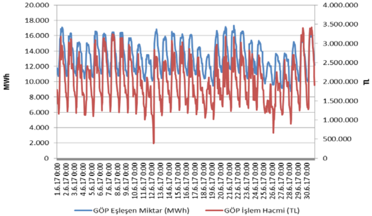
Şekil 4.2 Haziran 2017 Döneminde Gün Öncesi Piyasası (GÖP) İşlem Hacminin Saatlik Gelişimi (TL-MWh)
