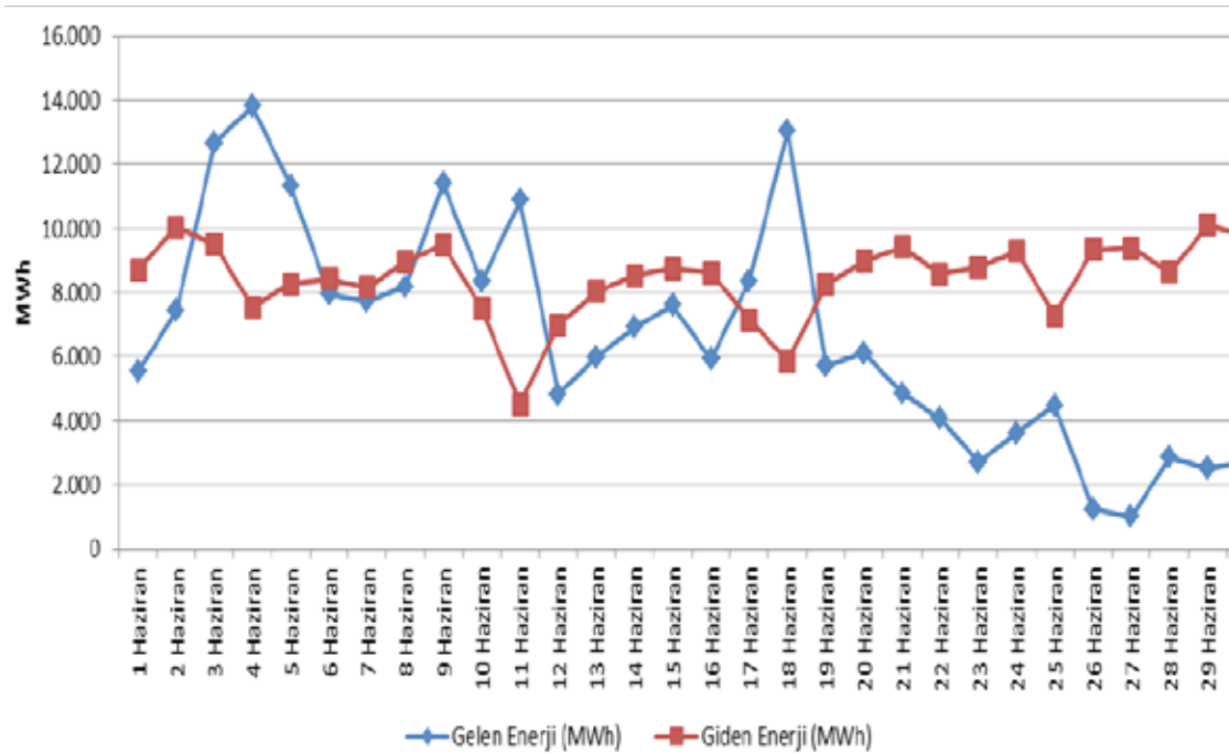
Şekil 3.1. Haziran 2017 Döneminde Günlük Bazda Yurtdışı Elektrik Ticareti (MWh)
