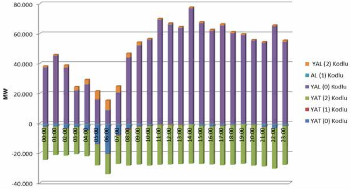
Şekil 4.7 Haziran 2017 Döneminde Dengeleme Güç Piyasasında (DGP) Verilen Talimatların Saatlik Bazda Dağılımı (MW)
