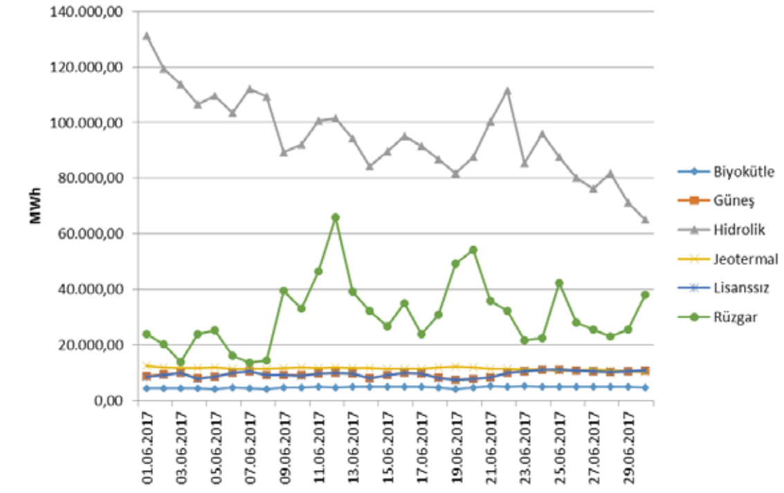
Şekil 1.12 Haziran 2017 Döneminde YEKDEM Kapsamındaki Üretimın Günlük Bazda Kaynaklara Göre Dağılımı (MWh)
