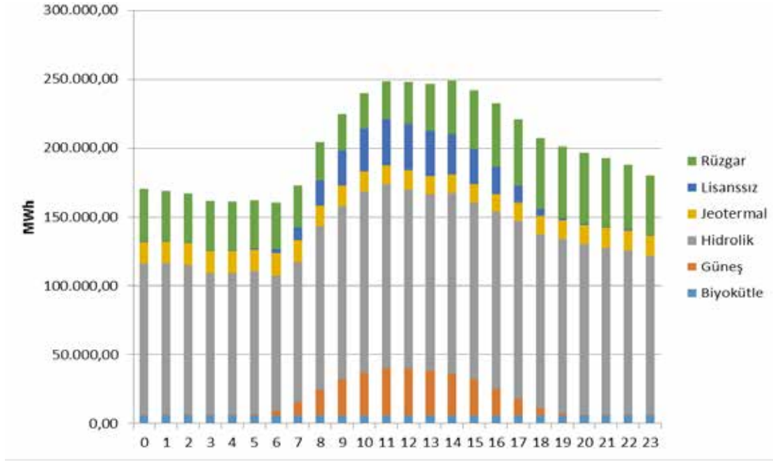
Şekil 1.11 Haziran 2017 Döneminde YEKDEM Kapsamındaki Üretimın Saatlik Bazda Kaynaklara Göre Dağılımı (MWh)
