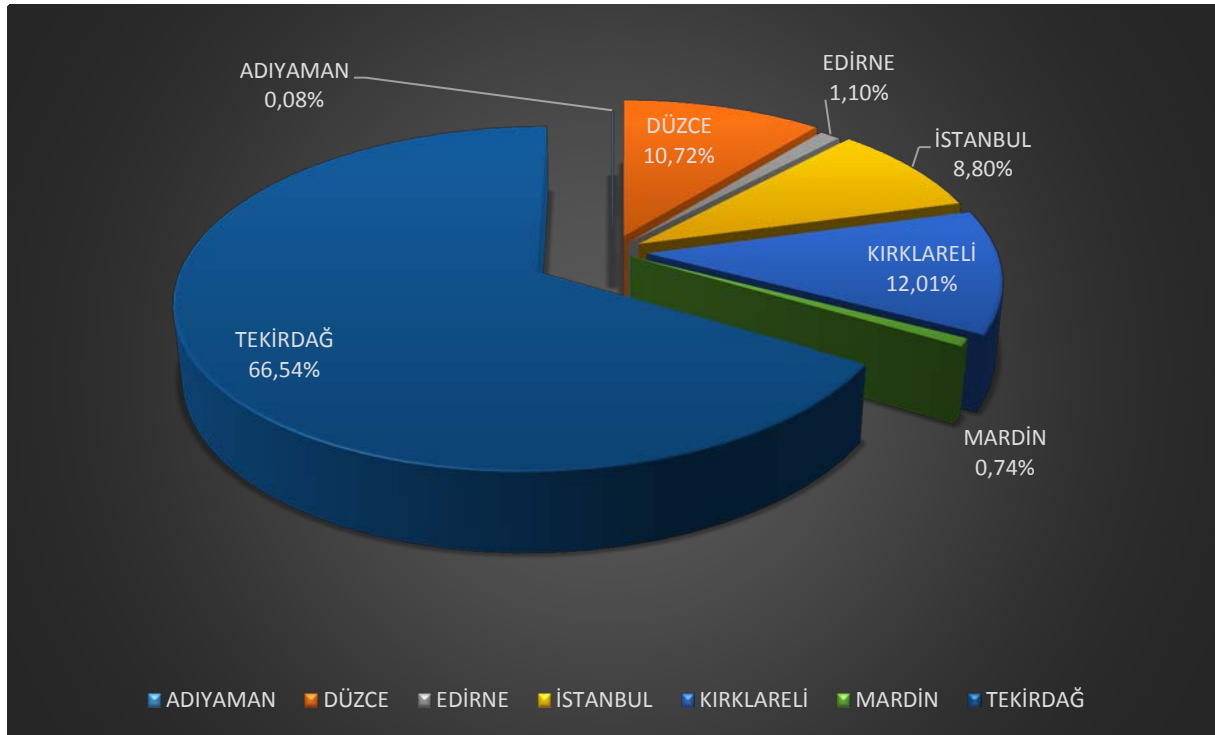
Grafik 1.1 2015 Ocak Ayında Üretim Sahalarının Bulunduğu İllere Göre Doğal Gaz Üretim Oranları (%)
