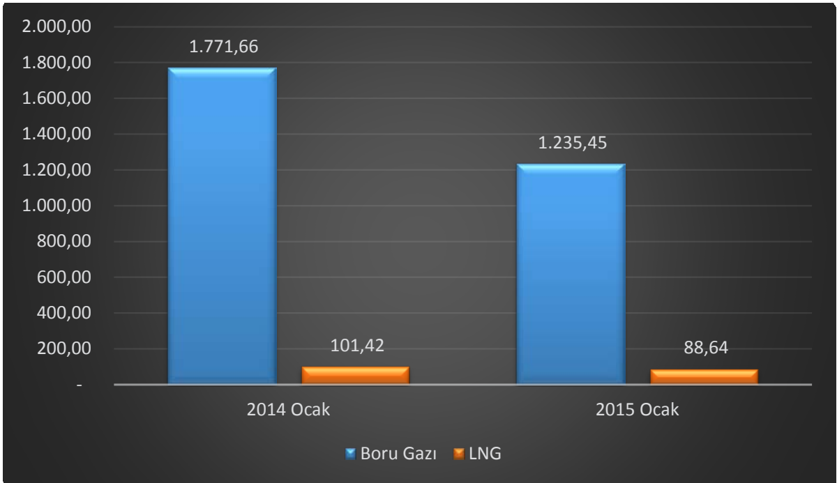
Grafik 3.1 Ocak 2014 ve Ocak 2015 Dönemlerindeki Depolama Stok Miktarlarının Gazın Türüne Göre Karşılaştırılması (Milyon Sm 3 )
