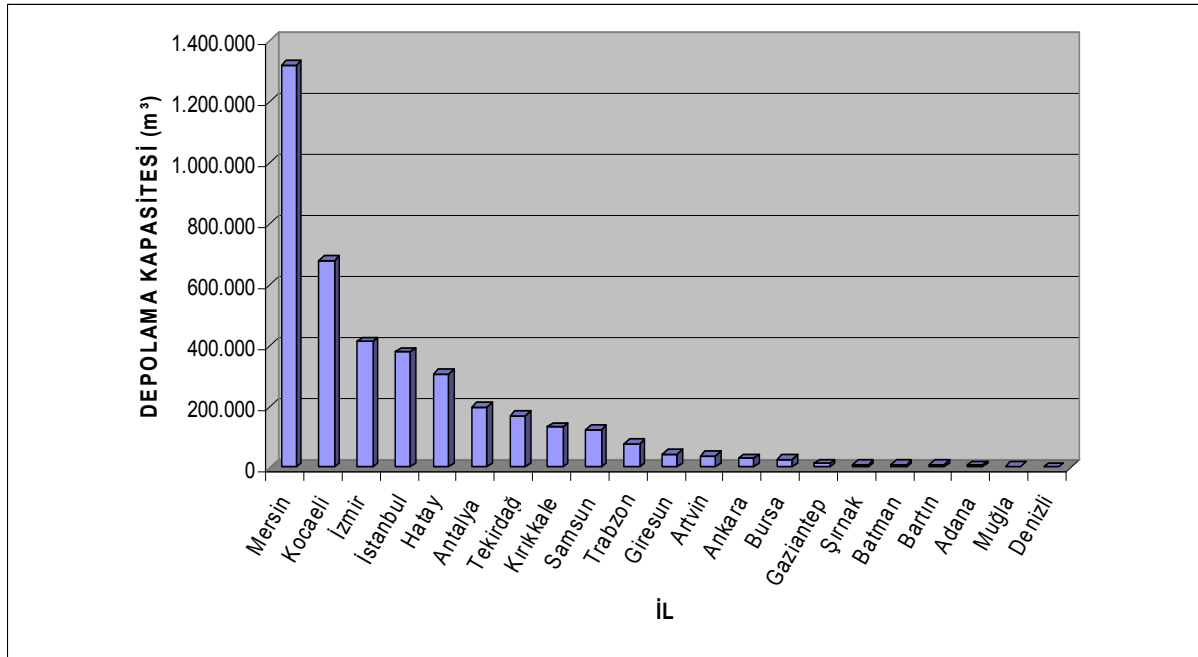
Grafik 9 - 2008 Sonu İtibarıyla Depolama Lisansı ve Depolama Alt Başlığı Kapsamındaki Depolama Kapasitelerinin İllere Göre Dağılımı
