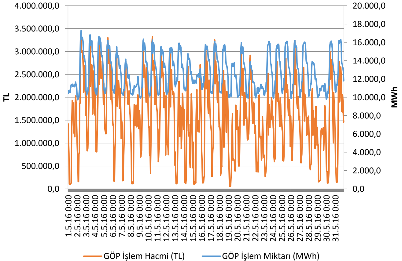
Grafik 4.2 Mayıs 2016 Döneminde Gün Öncesi Piyasası (GÖP)
