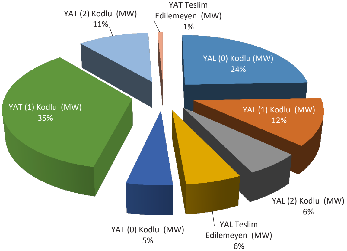
Grafik 4.4 Mayıs 2016 Döneminde Dengeleme Güç Piyasasında (DGP) Verilen Talimatların Oranı (%)
