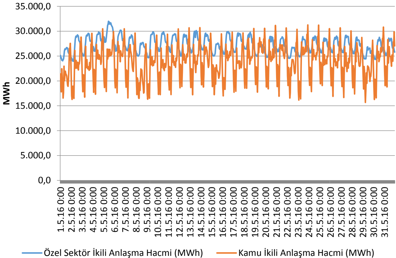
Grafik 4.6 Mayıs 2016 Döneminde İkili Anlaşma Hacminin Saatlik Gelişimi (MWh)
