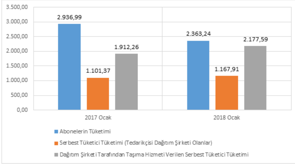
Şekil 5.4 Ocak 2018 Döneminde Doğal Gaz Dağıtım Bölgelerindeki Toplam Boru Gazı Tüketim Miktarı (Milyon Sm 3 )
