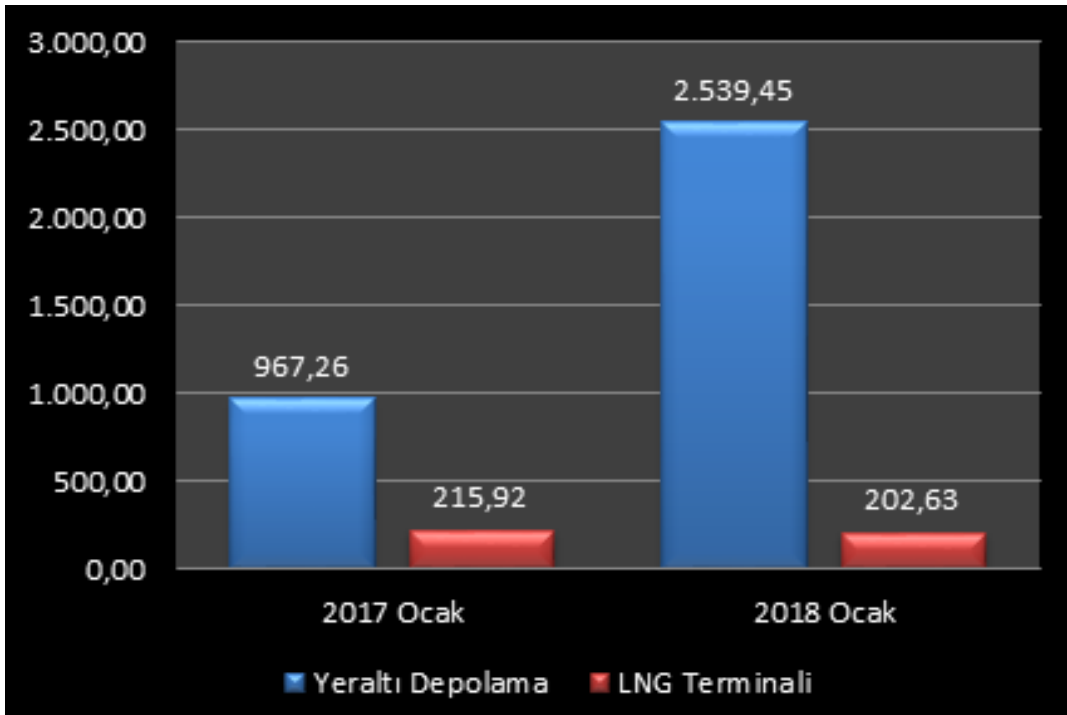
Şekil 3.1 Ocak 2017 ve Ocak 2018 Dönemlerindeki Depolama Stok Miktarlarının Depolama Türüne Göre Karşılaştırılması (Milyon Sm 3 )
