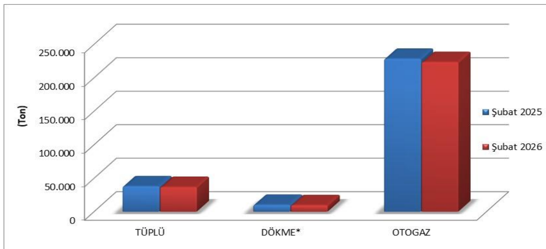
Şekil 3.2: Şubat 2025 – Şubat 2026 Dönemlerinde Ürün Türüne Göre LPG Satışları
