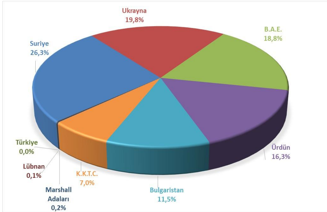
Şekil 2.2: Şubat 2026 Dönemi LPG İhracatının Ükelere Göre Dağılımı
