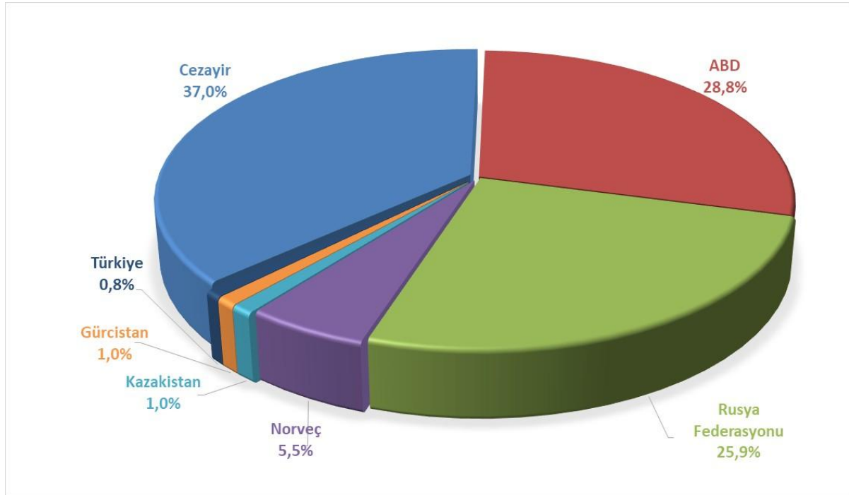
Şekil 2.1: Şubat 2026 Dönemi LPG İthalatının Ülkelere Göre Dağılımı
