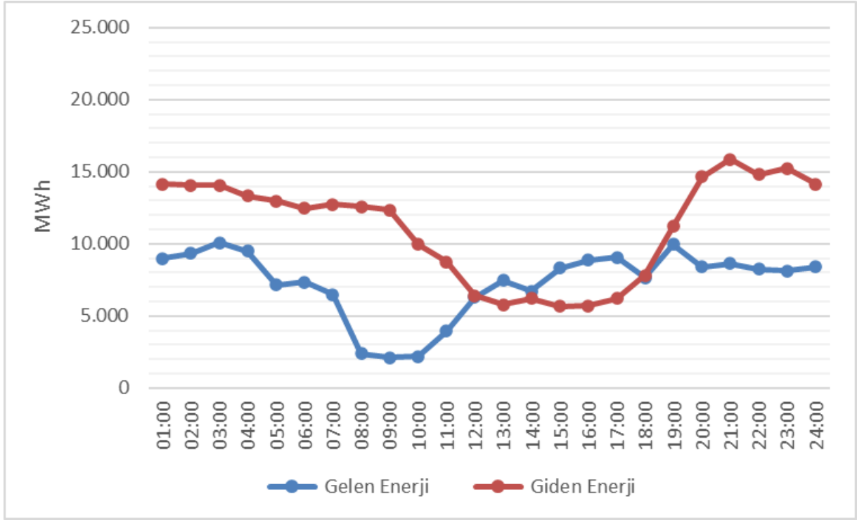
Şekil 3.2 Temmuz 2026 Döneminde Saatlik Bazda Yurtdışı Elektrik Ticareti (MWh)
