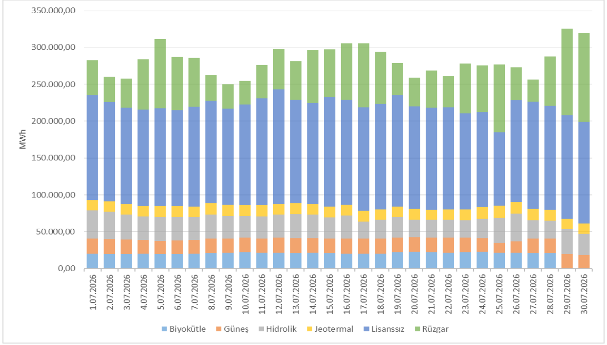
Şekil 1.11 Temmuz 2026 Döneminde YEKDEM Kapsamındaki Üretimin Günlük Bazda Kaynaklara Göre Dağılımı (MWh)
