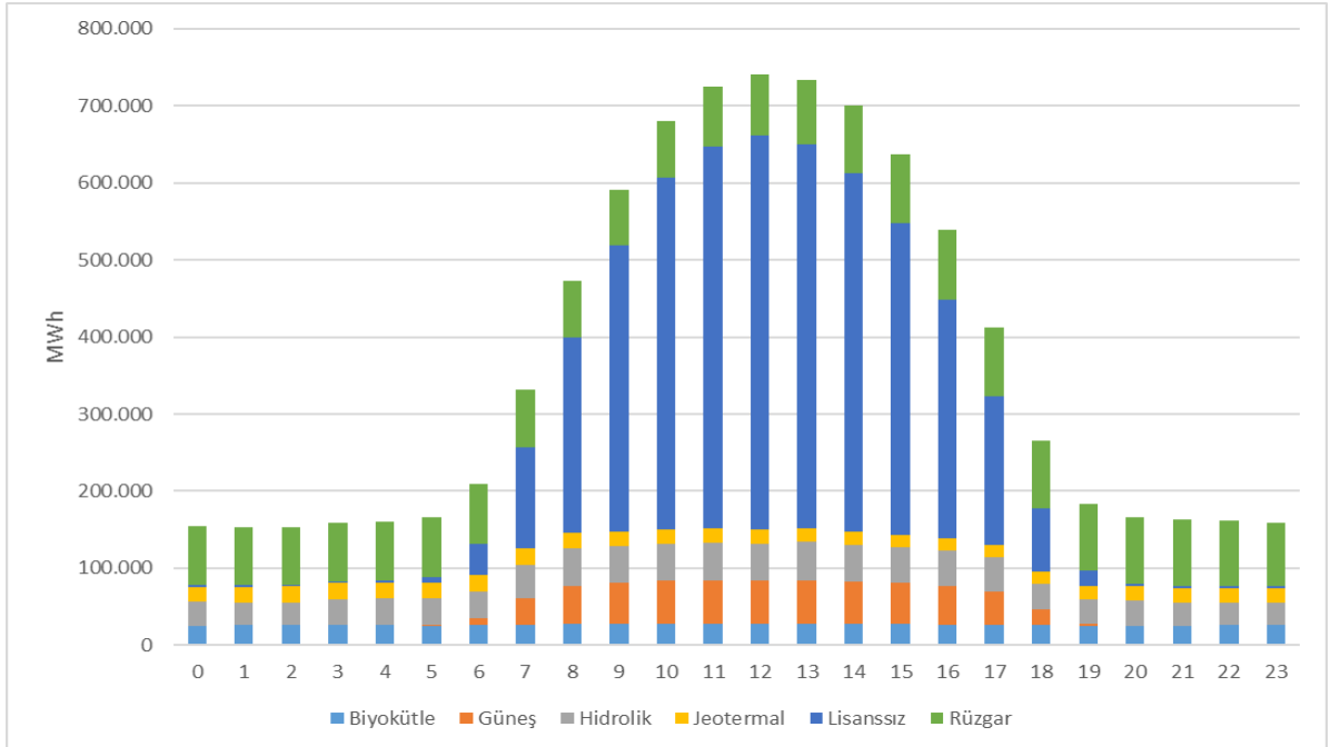
Şekil 1.10 Temmuz 2026 Döneminde YEKDEM Kapsamındaki Üretimin Saatlik Bazda Kaynaklara Göre Dağılımı (MWh)
