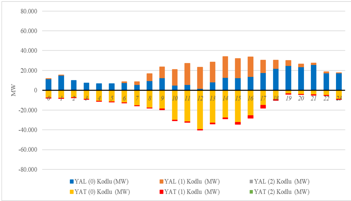
Şekil 4.7 Temmuz 2026 Döneminde Dengeleme Güç Piyasasında (DGP) Verilen Talimatların Saatlik Bazda Dağılımı (MW)
