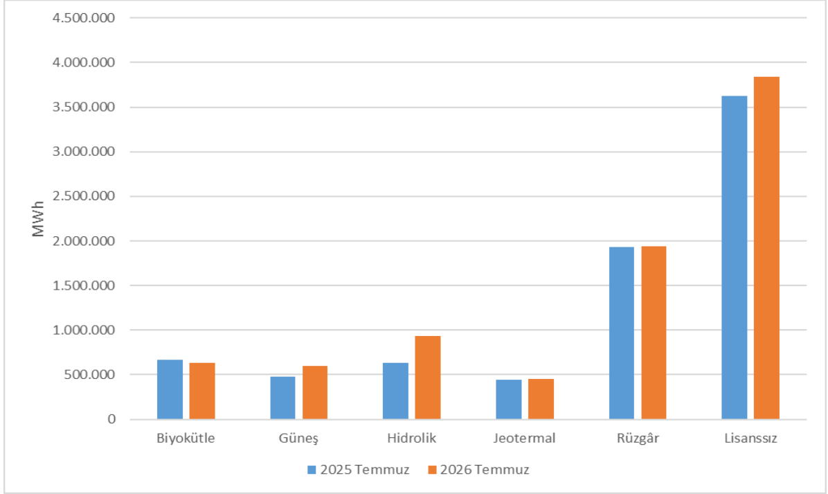
Şekil 1.9 2025-2026 Temmuz Dönemi YEKDEM Kapsamındaki Üretimin Kaynaklara Göre Dağılımı
