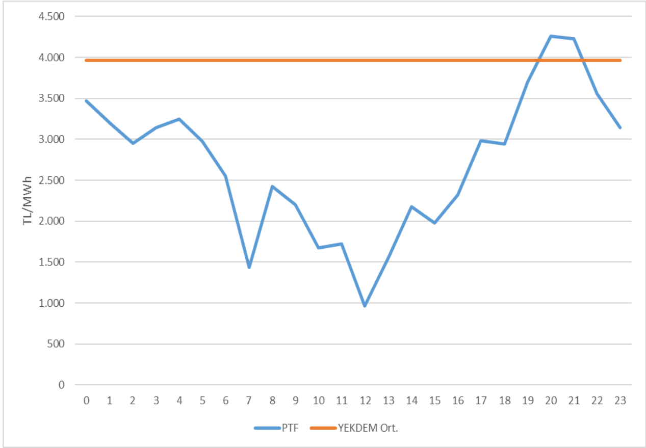
Şekil 1.12 Temmuz 2026 Döneminde YEKDEM Aylık Ortalama Fiyatı ile Piyasa Takas Fiyatının (PTF) Saatlik Dağılımı (TL/MWh)
