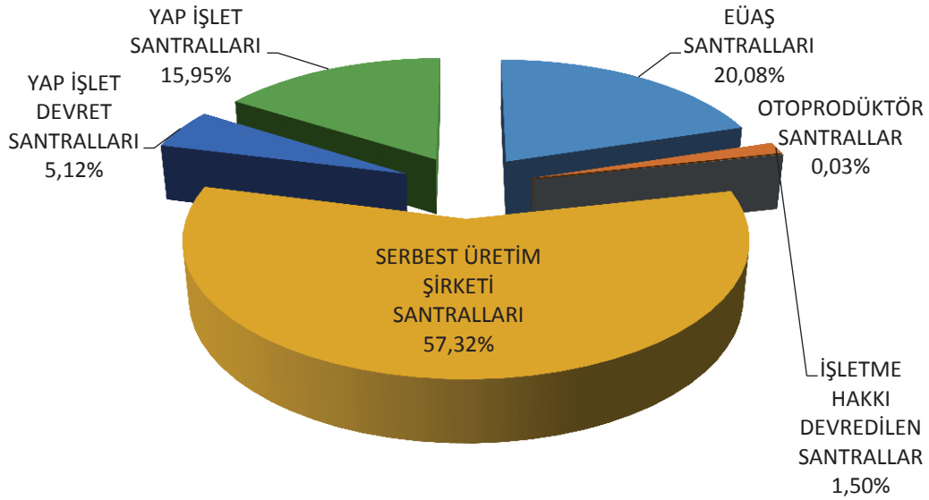
Grafik 1.3 Ocak 2016 Döneminde Elektrik Üretimine Kuruluş Bazında Dağılım Oranları (%)
