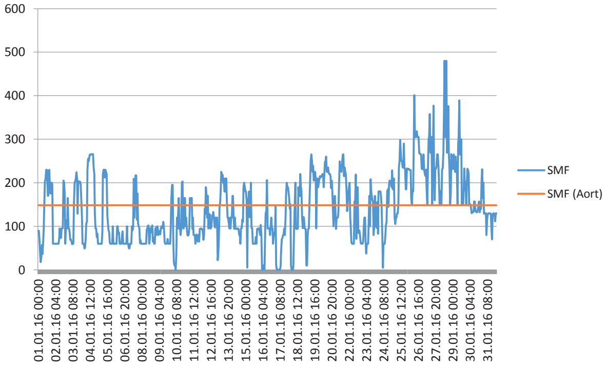
Grafik 4.2 Ocak 2016 Döneminde Sistem Marjinal Fiyatının(SMF) Gelişimi (TL/MWh)
