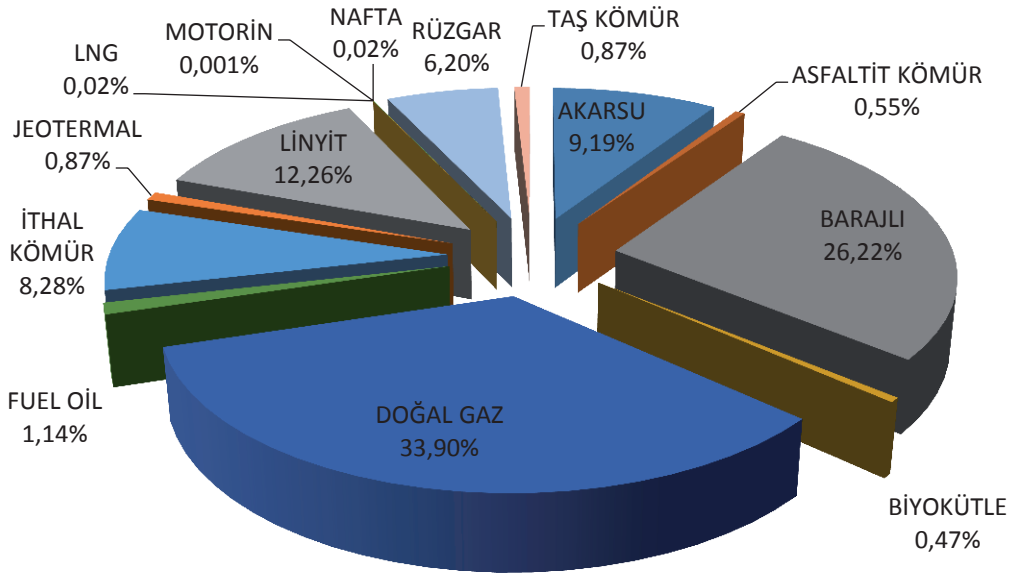
Grafik 1.2 2016 Yılı Ocak Ayı Sonu İtibariyle Kurulu Gücün Kaynak Bazında Dağılımı (%)
