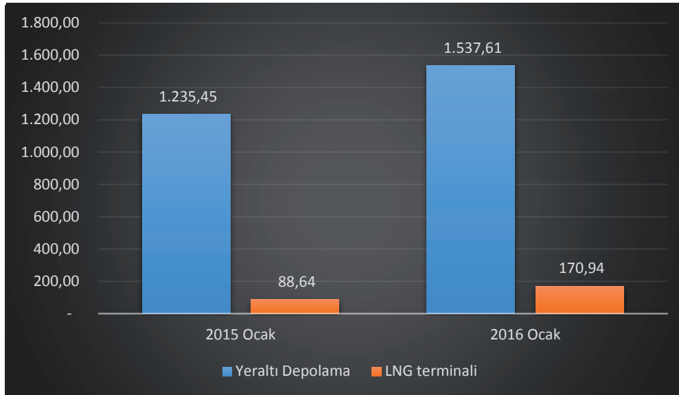
Grafik 3.1 Şubat 2015 ve Şubat 2016 Dönemlerindeki Depolama Stok Miktarlarının Depolama Türüne Göre Karşılaştırılması (Milyon Sm 3 )
