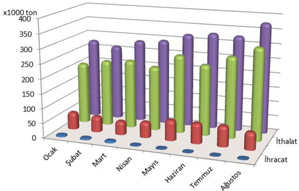
Şekil 4.1.1: Aylık LPG üretim-satış-ithalat-ihracat miktarları
